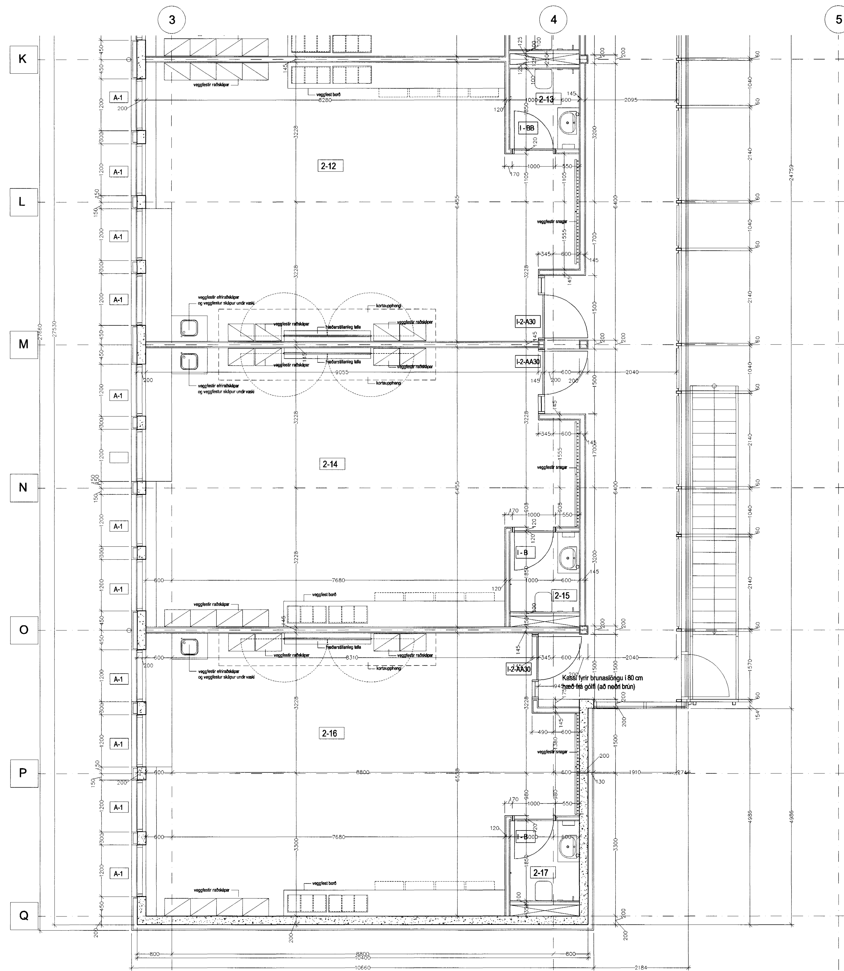
GRUNNMYND 2. HÆÐAR 1:50, ÞVERÁLMA
