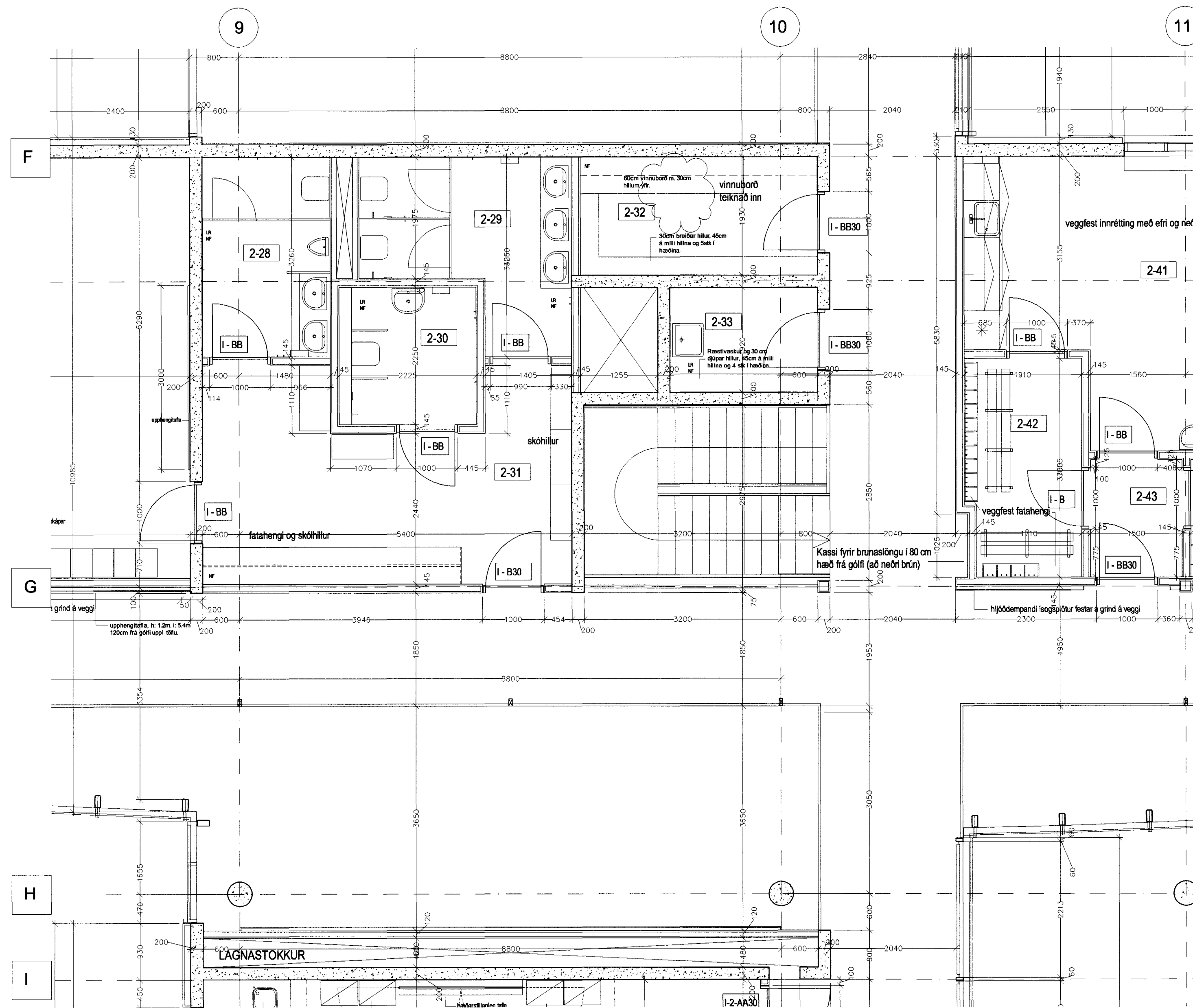
GRUNNMYND 2. HÆÐAR 1:50, ADALÁLMA
