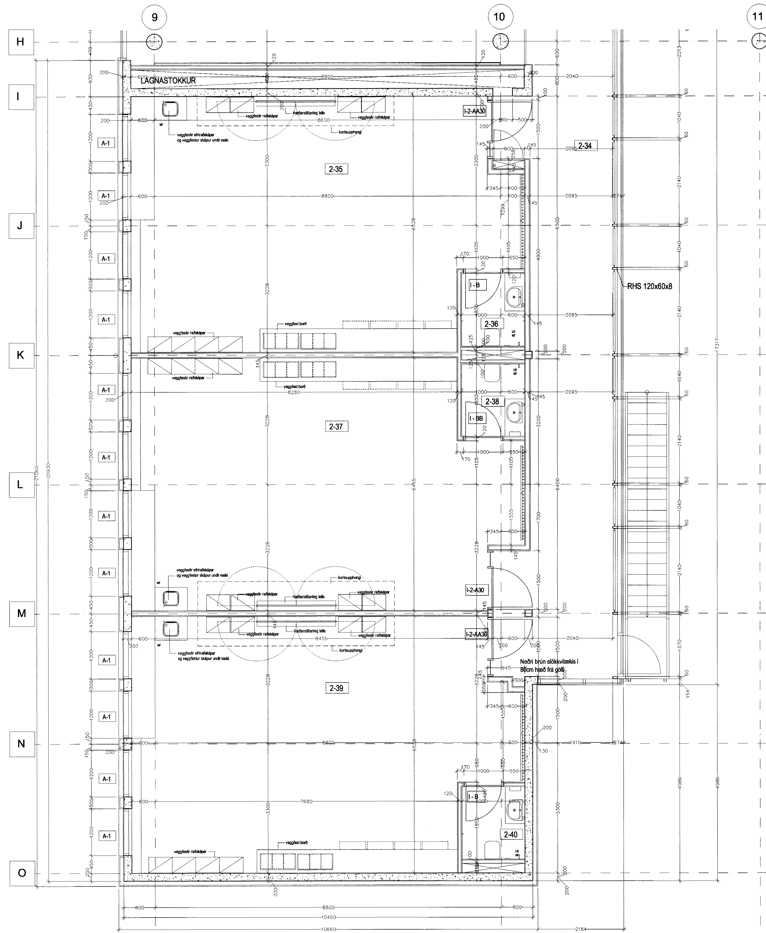
GRUNNMYND 2. HÆÐAR 1:50, ÞVERÁLMA
