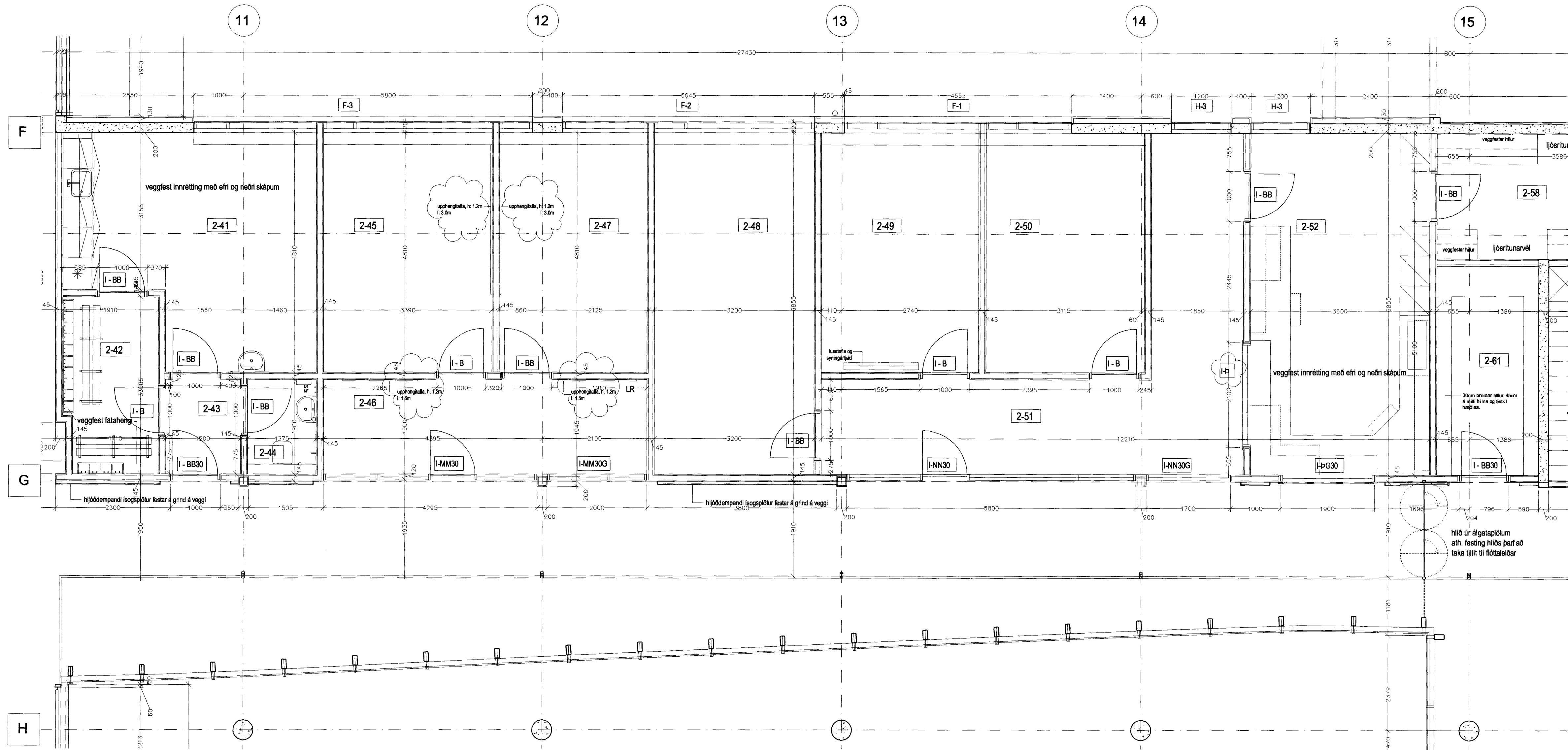
GRUNNMYND 2. HÆÐAR 1:50, ADALÁLMA
