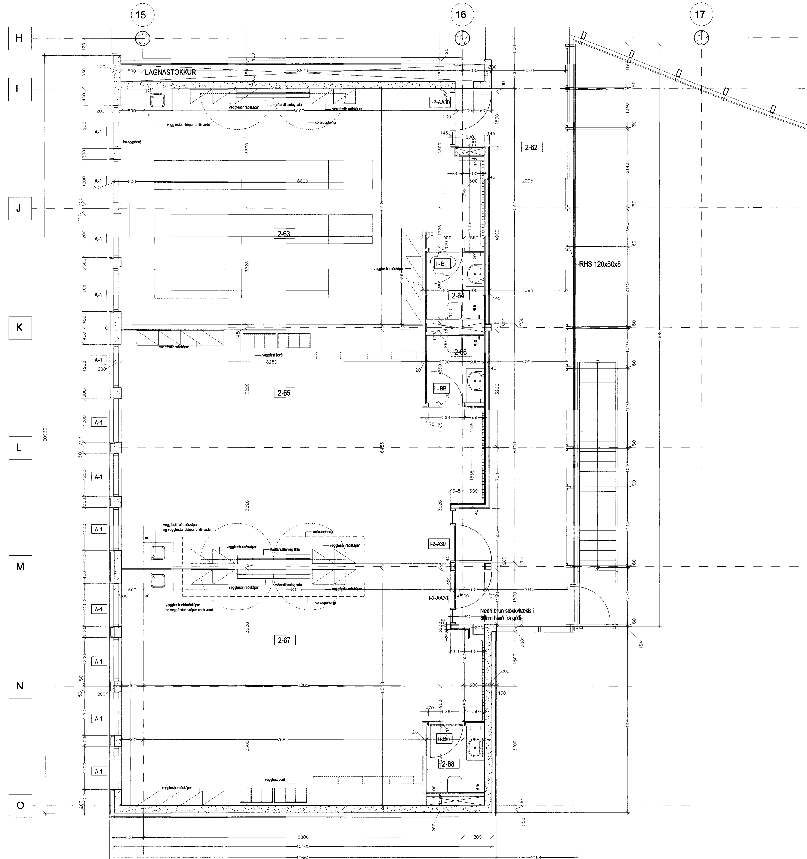
GRUNNMYND 2. HÆÐAR 1:50, ÞVERÁLMA
