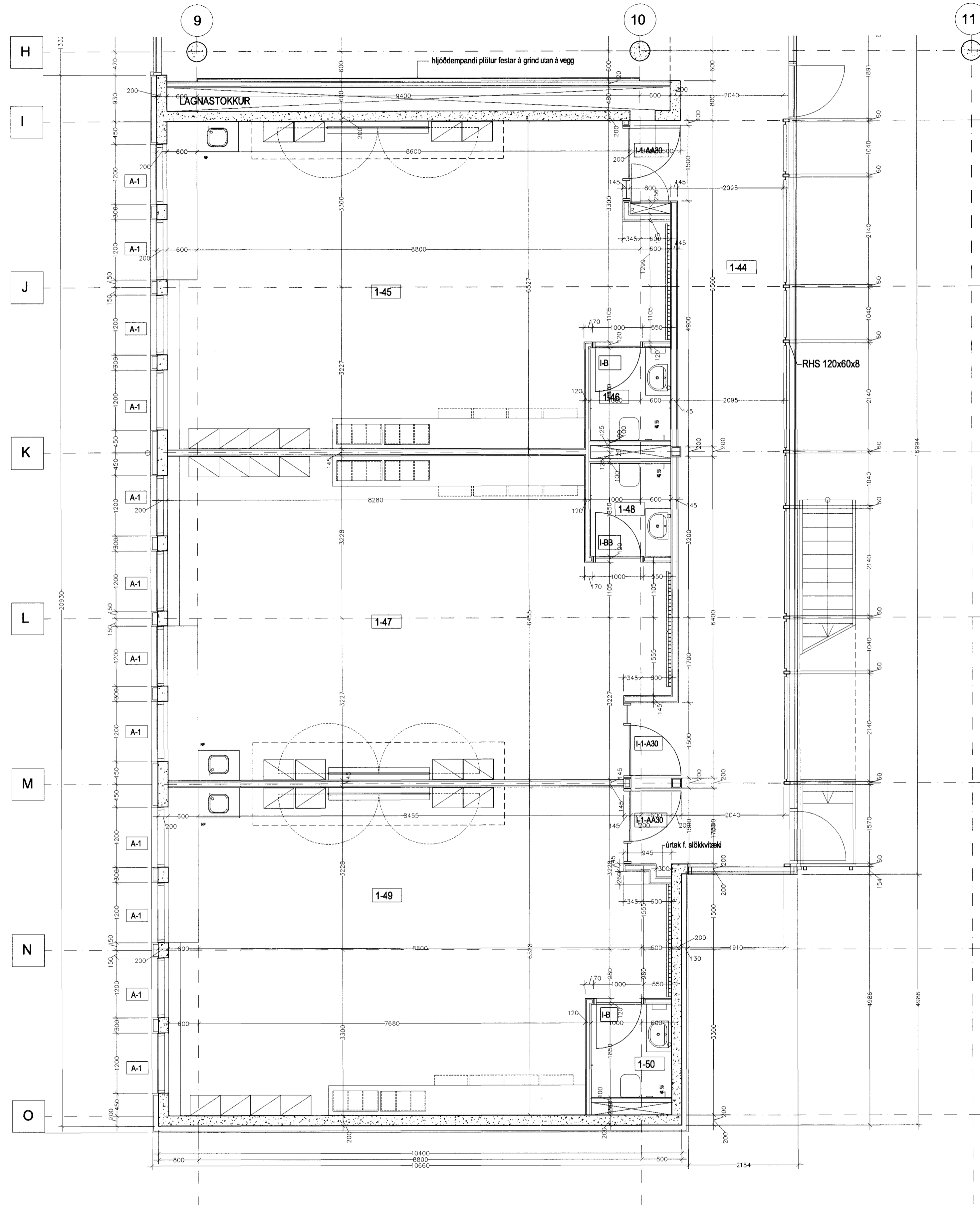
GRUNNMYND 1. HÆÐAR 1:50, ÞVERÁLMA
