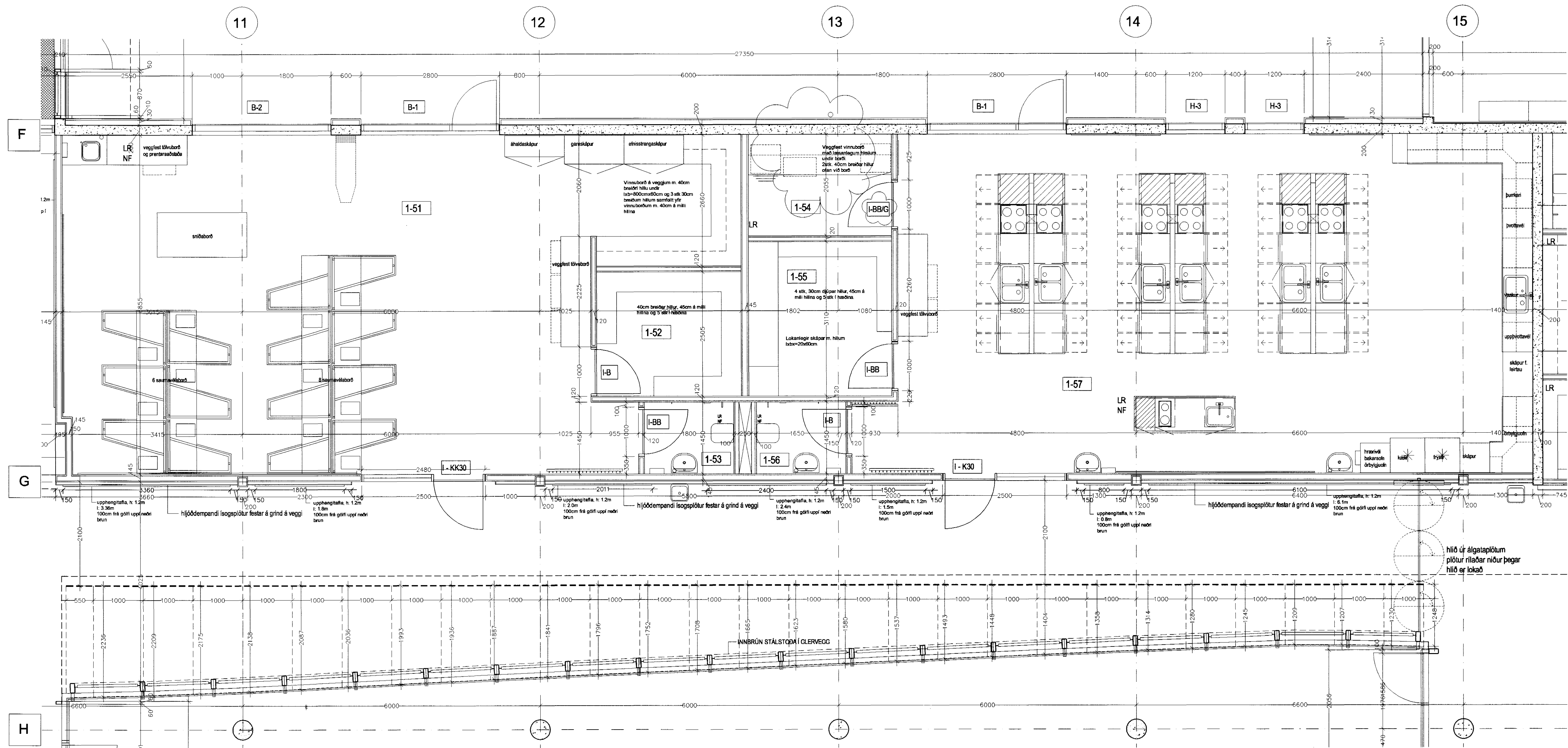
GRUNNMYND 1. HÆÐAR 1:50, AÐALÁLMA
