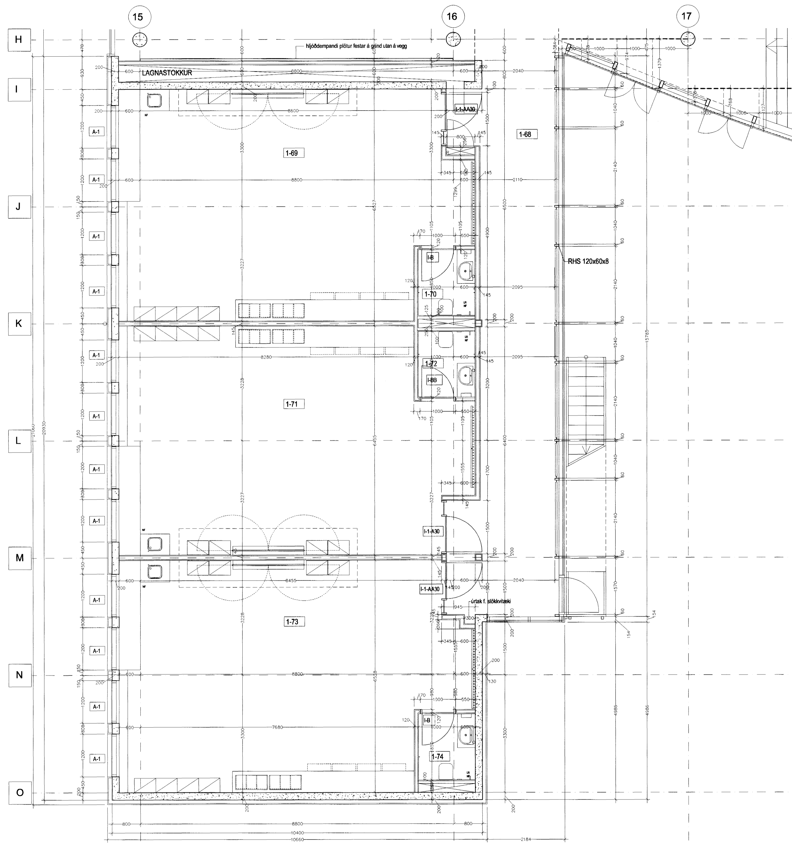
GRUNNMYND 1. HÆÐAR 1:50, ÞVERÁLMA
