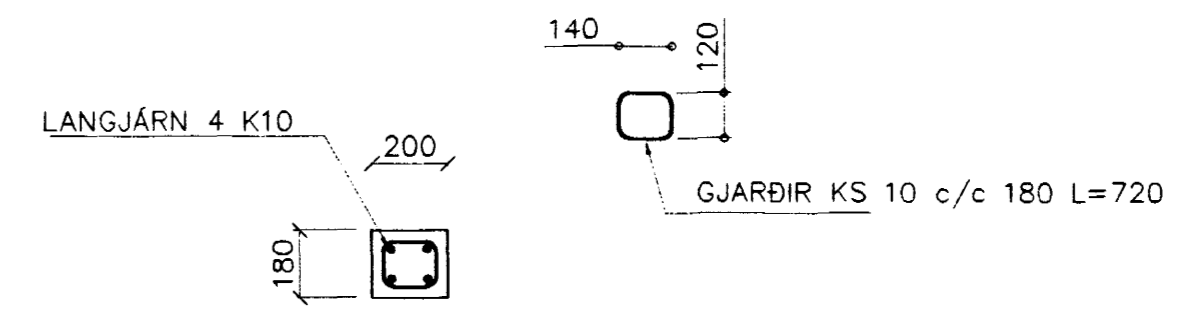
SÚLA S1 1:20
