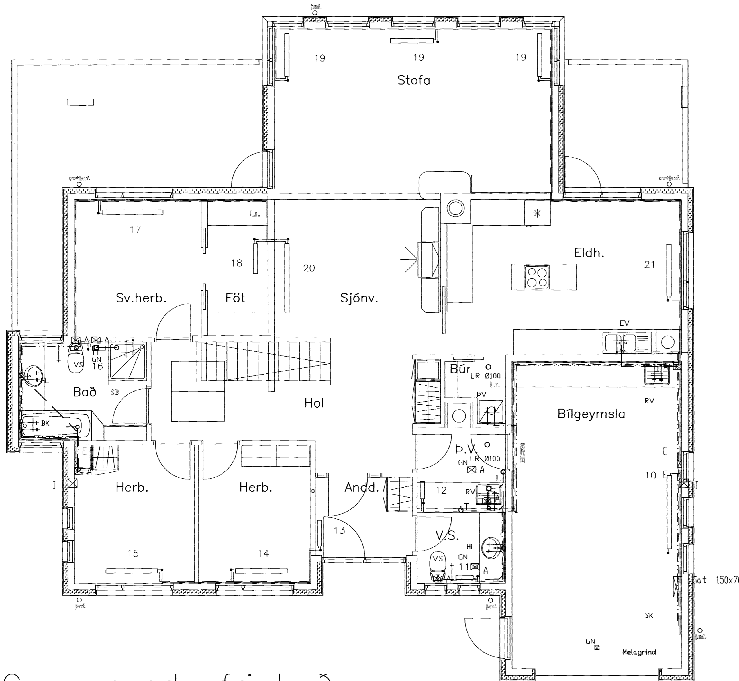
Grunnmynd efri hæð
