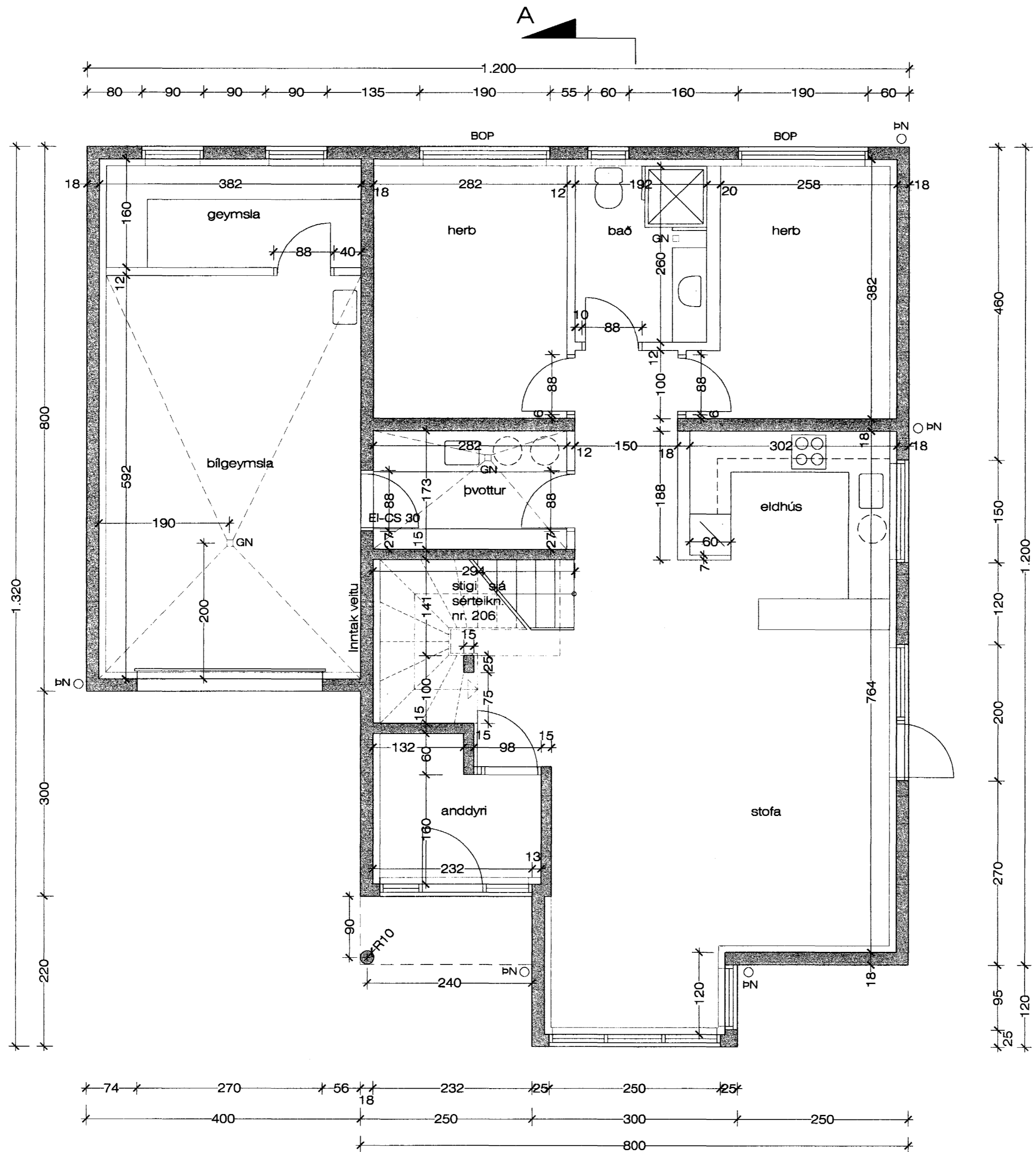
GRUNNMYND NEDRI HÆÐ M 1 : 50
