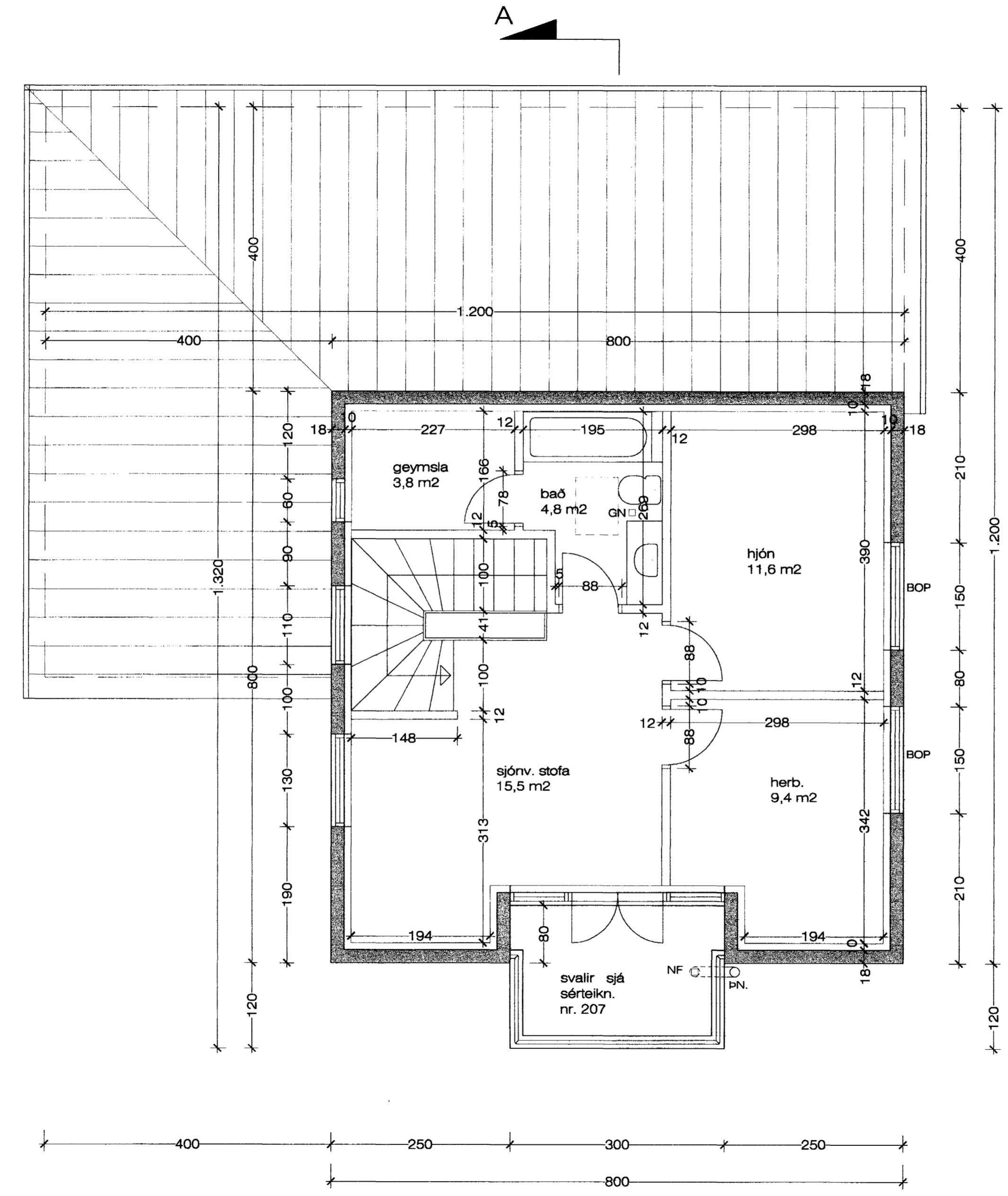
GRUNNMYND EFRI HÆÐ M 1 : 50
