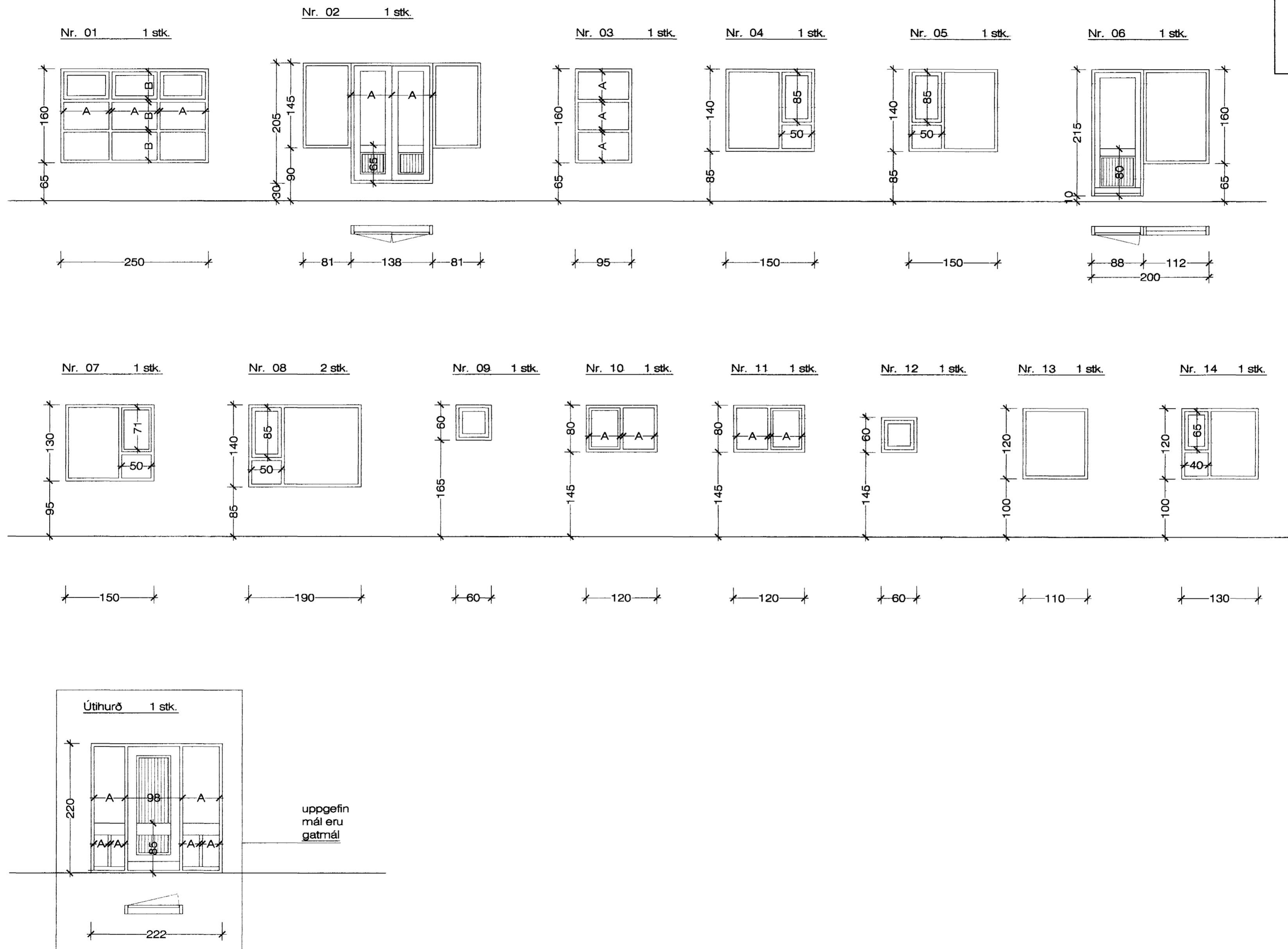
GLUGGAR OG HURÐIR M 1 : 50
