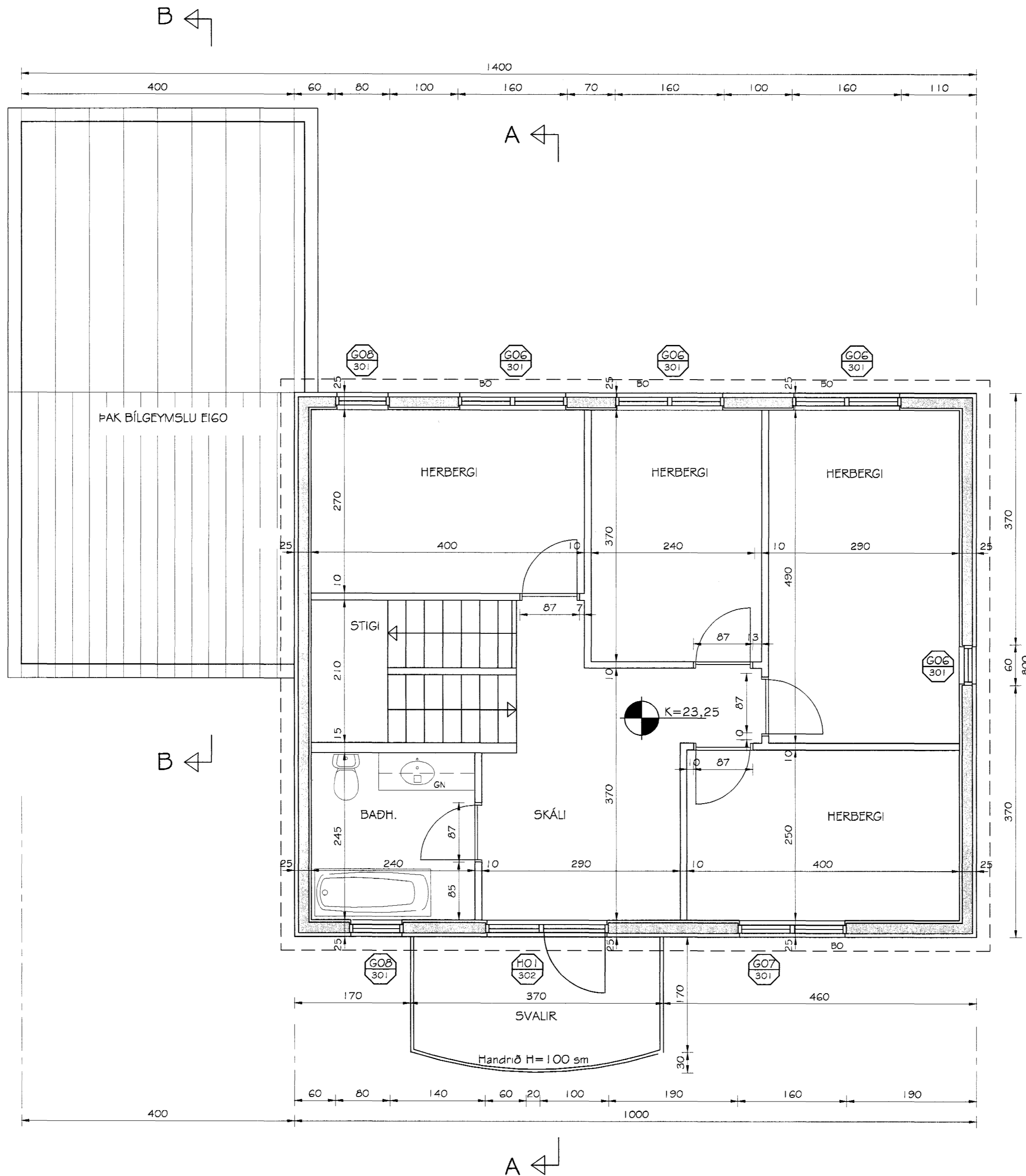
GRUNNMYND EFRÍ HÆÐAR MKV. 1:50
