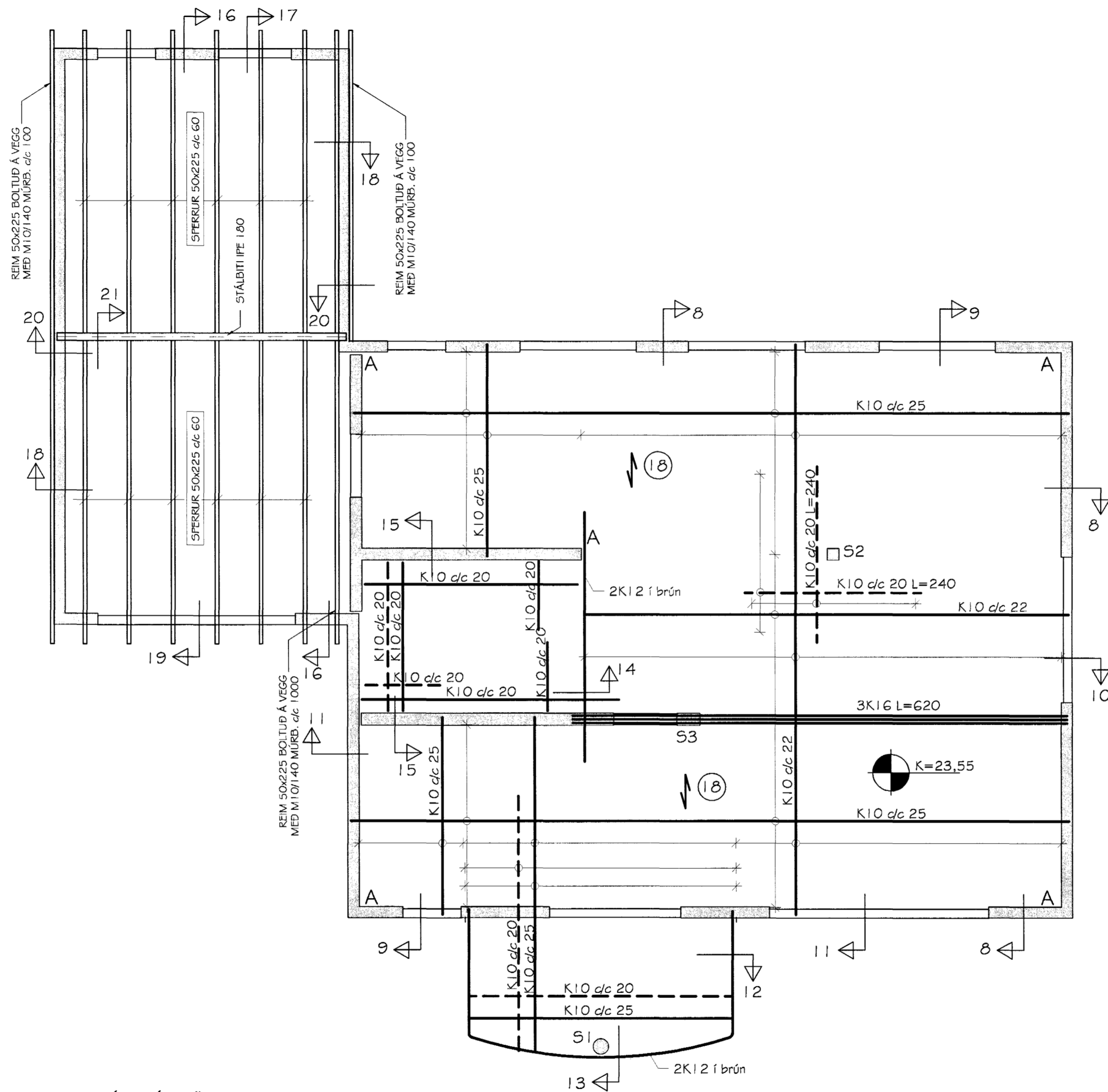
JÁRN Í PLÖTU YFIR NEDRI HÆÐ ÞAKVIÐIR YFIR BÍLGEYMSLU GRUNNMYND MKV. 1:50
