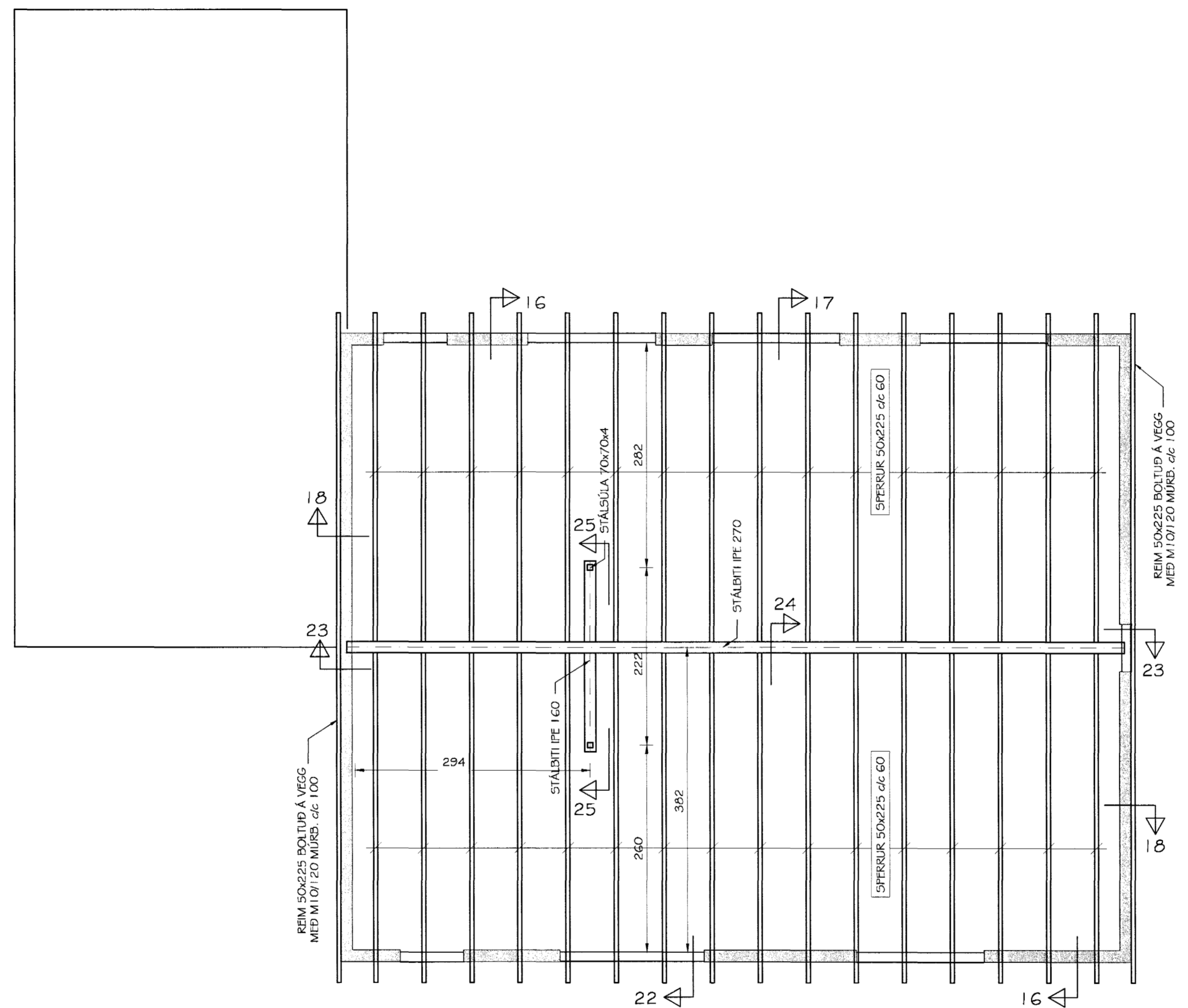
GRUNNMYND ÞAKVIÐA MKV. 1:50
