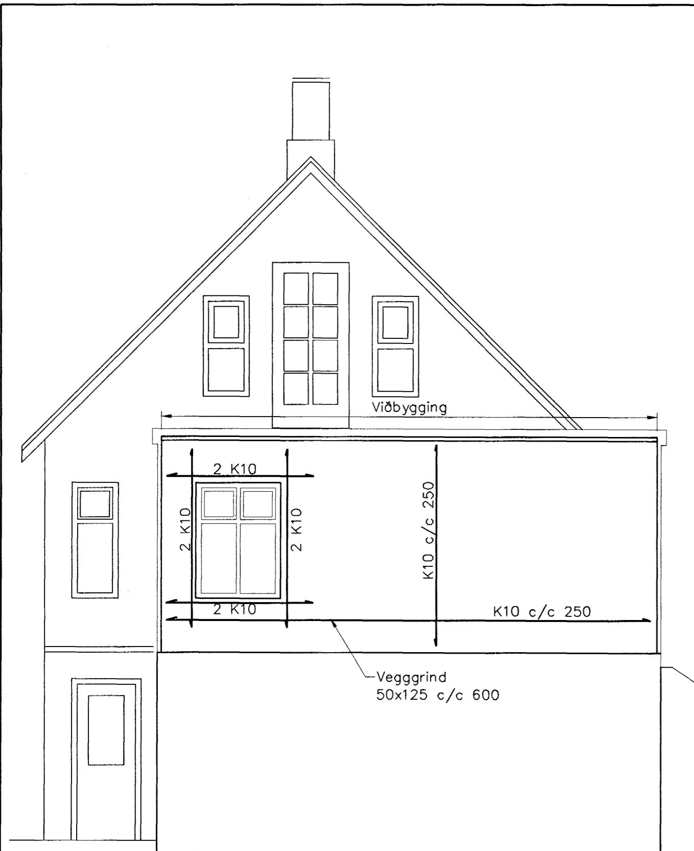
Ásýnd suður, 1:50
