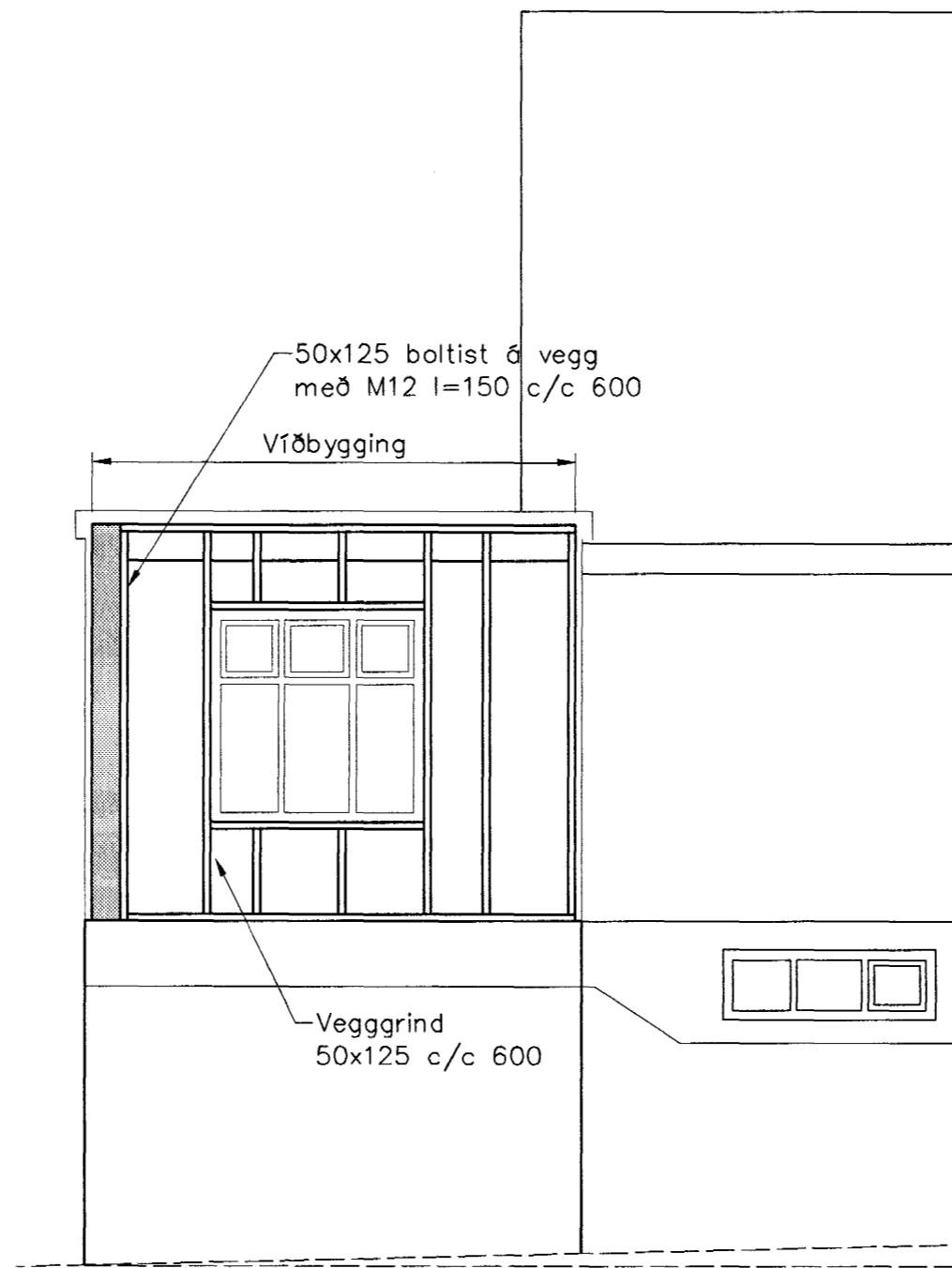
Ásýnd austur, 1:50
