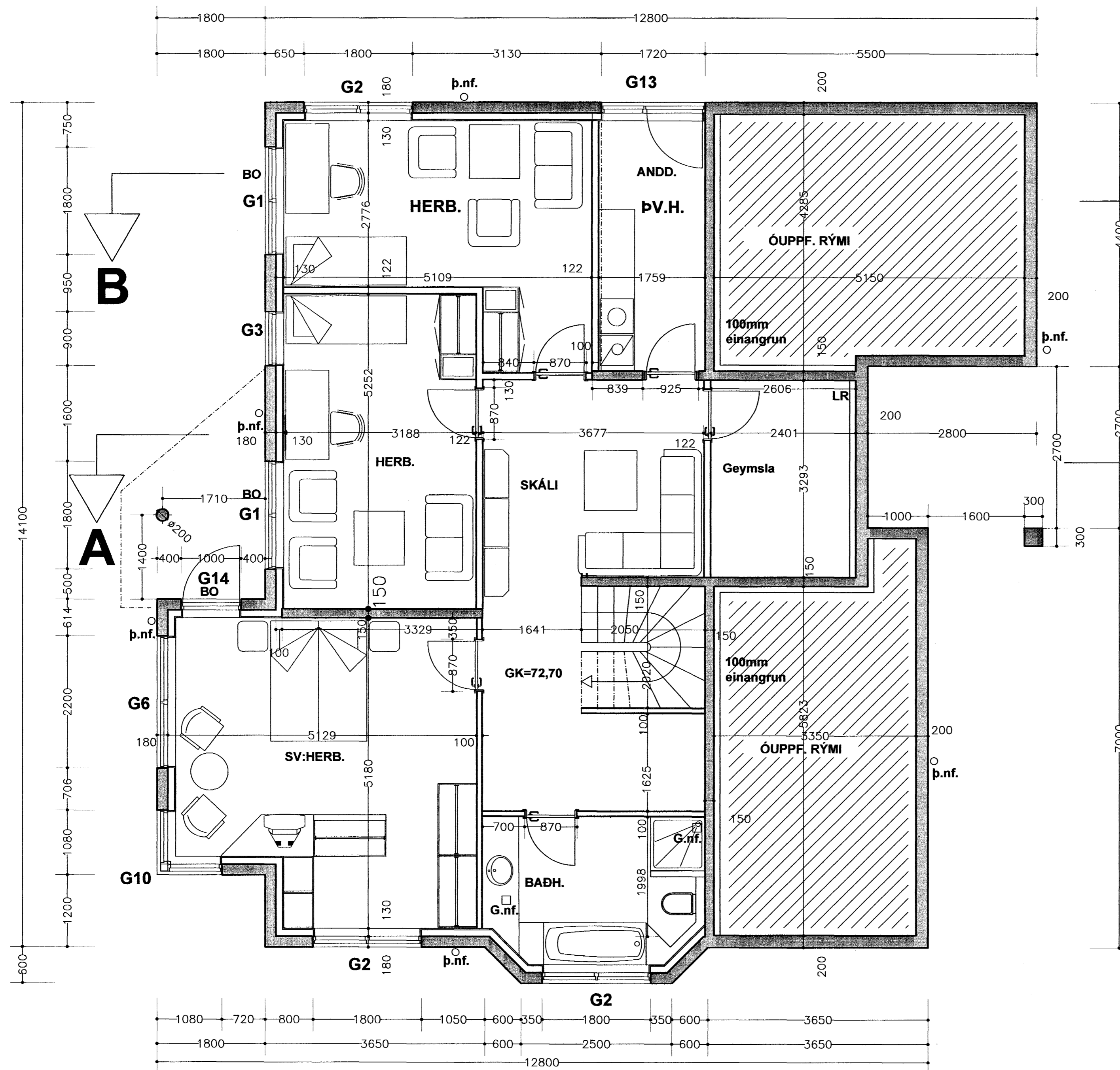
Grunnmynd 1. hæð
