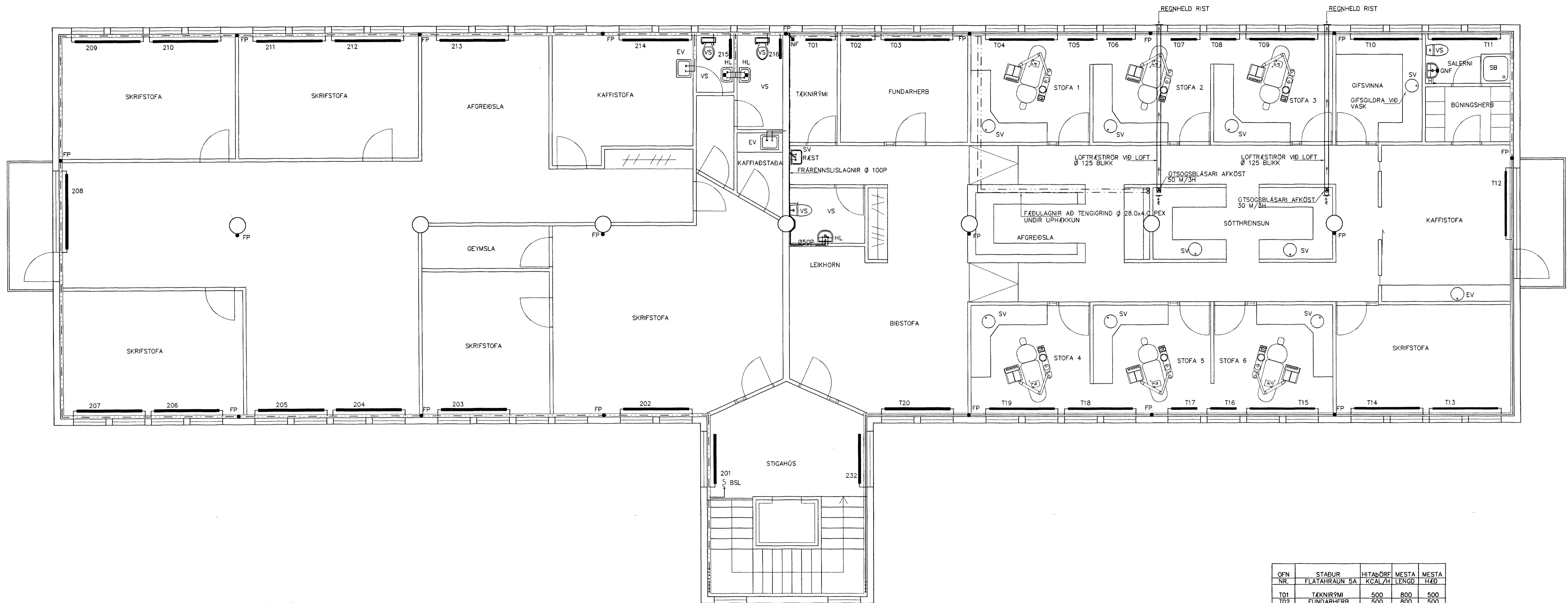
GRUNNMYND 2 HÆÐAR 1:50
