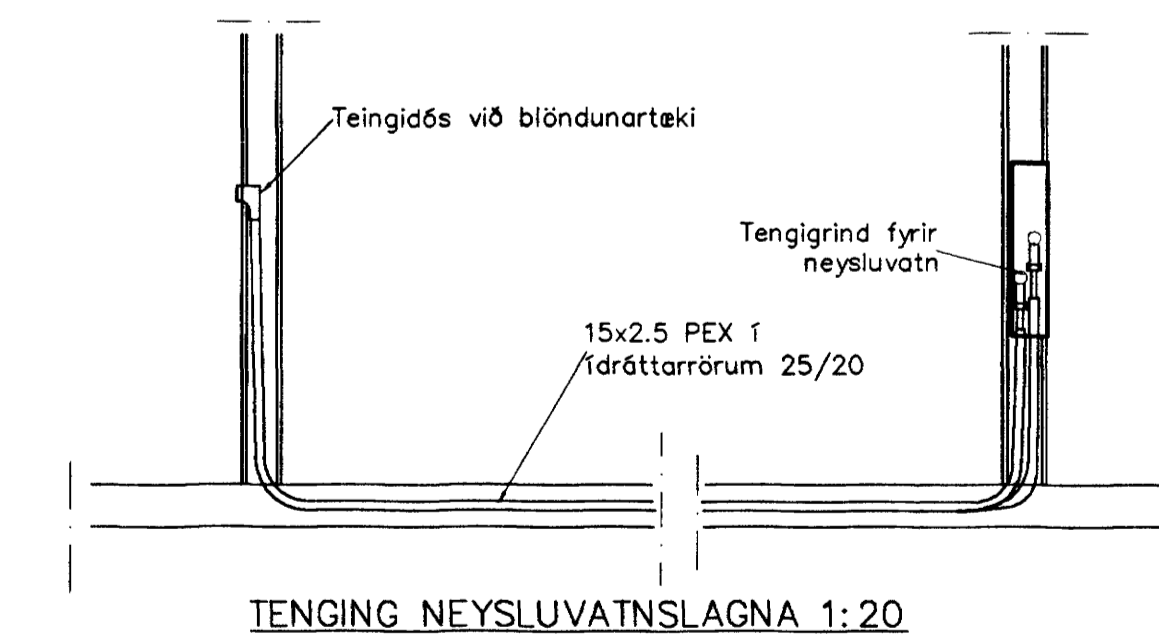
TENGING NEYSLUVATNSLAGNA 1:20
