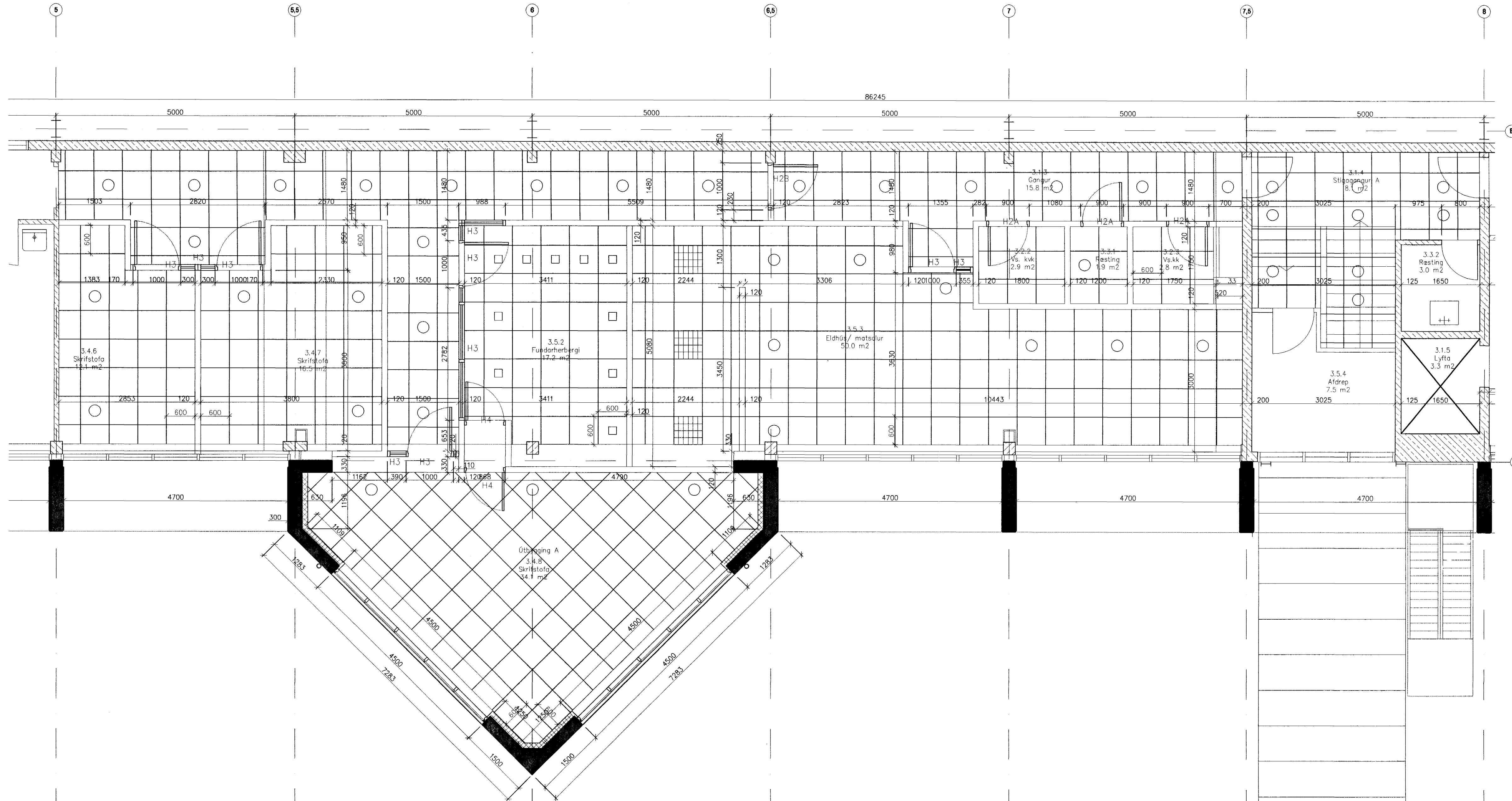
(45)3.02 Loftaplan 3. hæð skrifstofulíma (partur) Málkvarði 1:50
