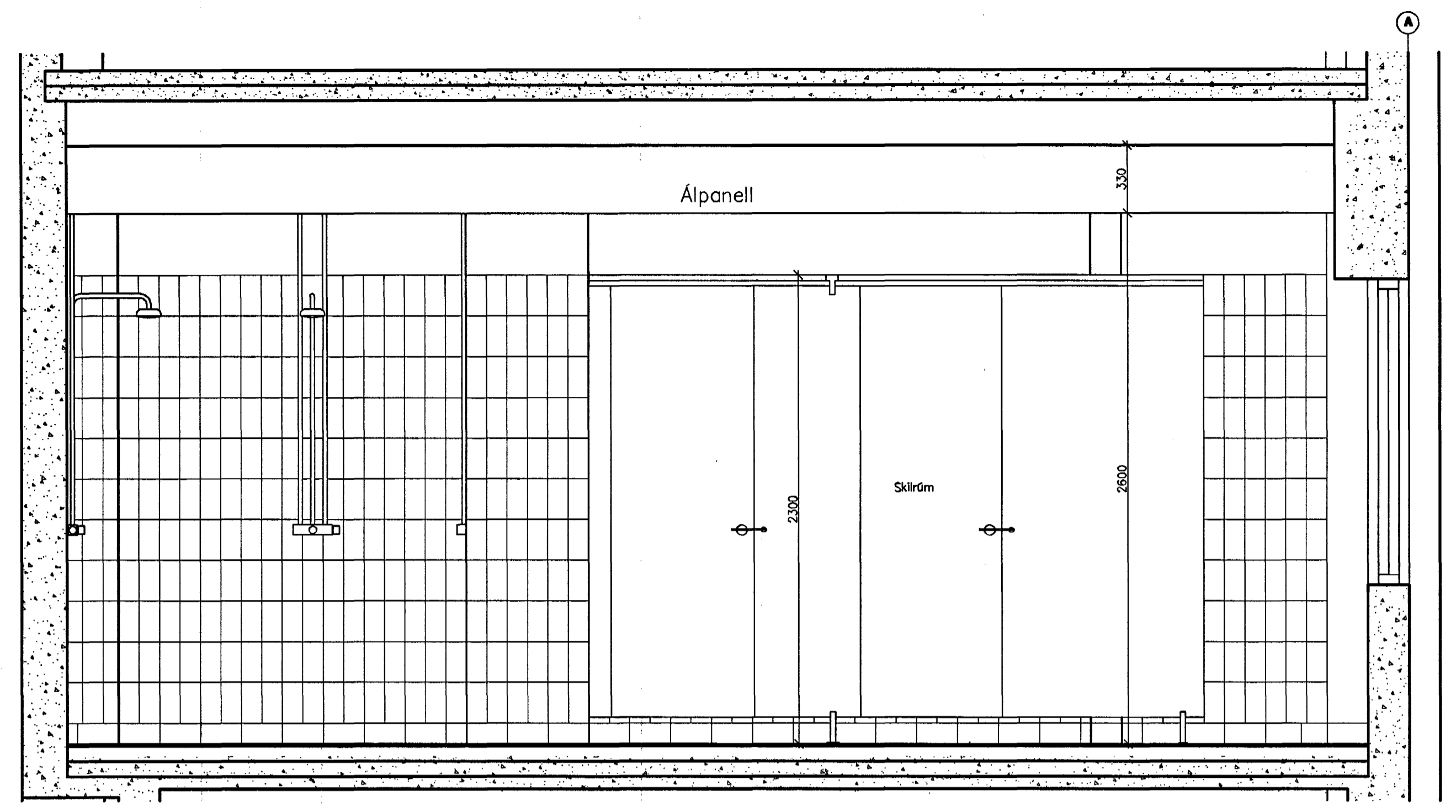
(79)A.11.11. Búningaklefi (partur), þvallasæði og snýringar - 2h. Sneiðing F-F
