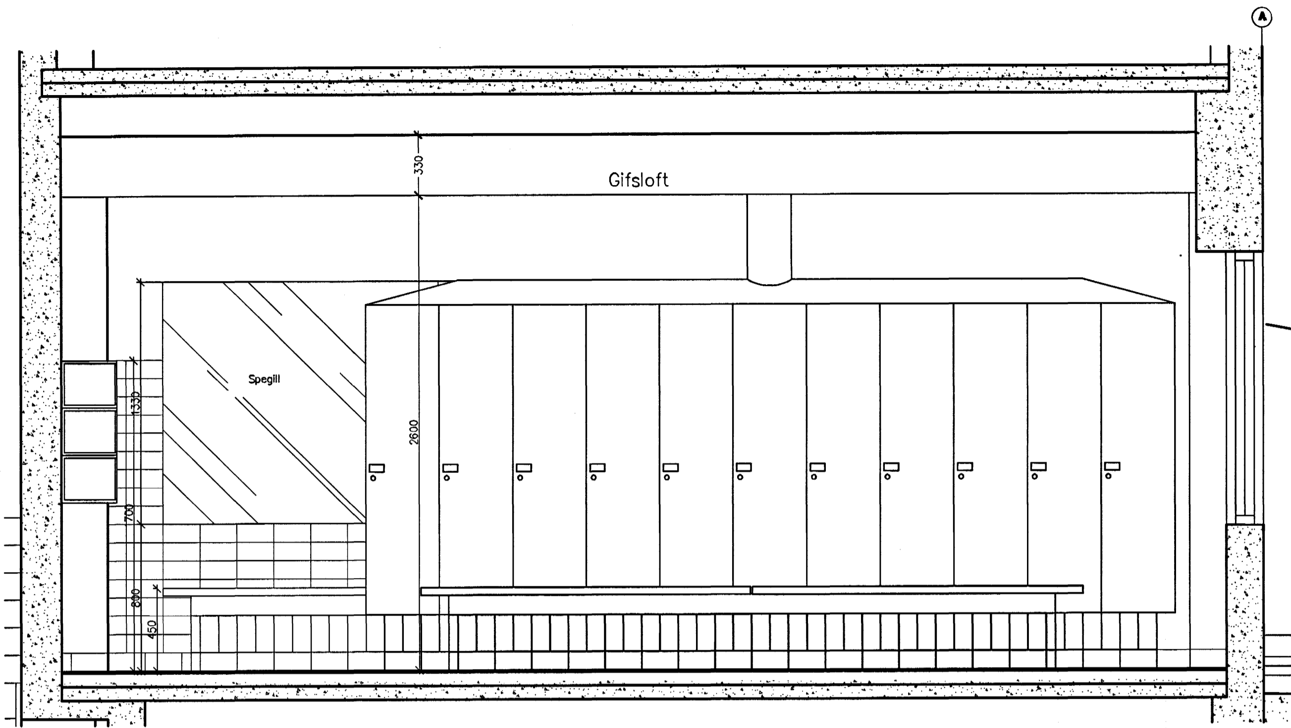
(79)A.11.11. Búningaklefi (partur), þvallasæði og snýringar - 2h. Sneiðing E-E
