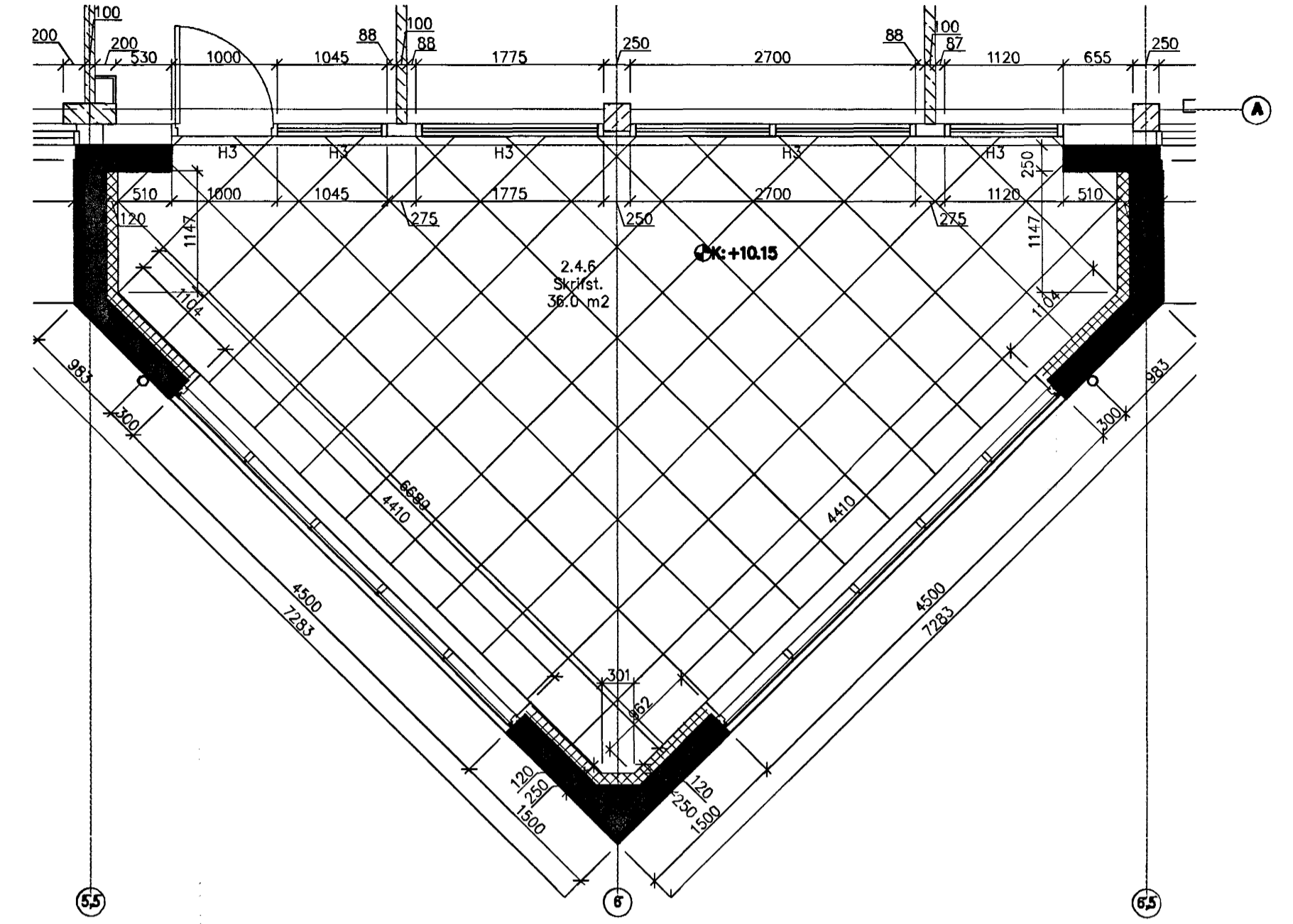
(43)3.01 Gólfefni 2h - vöbýgging skrifstofu
