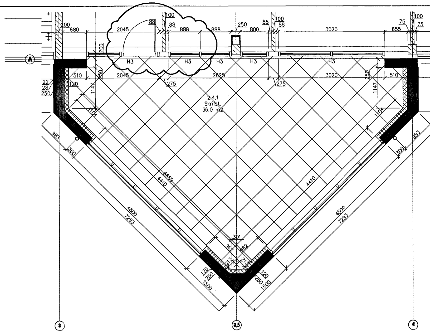
(43)3.01 Gólfefni 2h - vöbýgging skrifstofu
