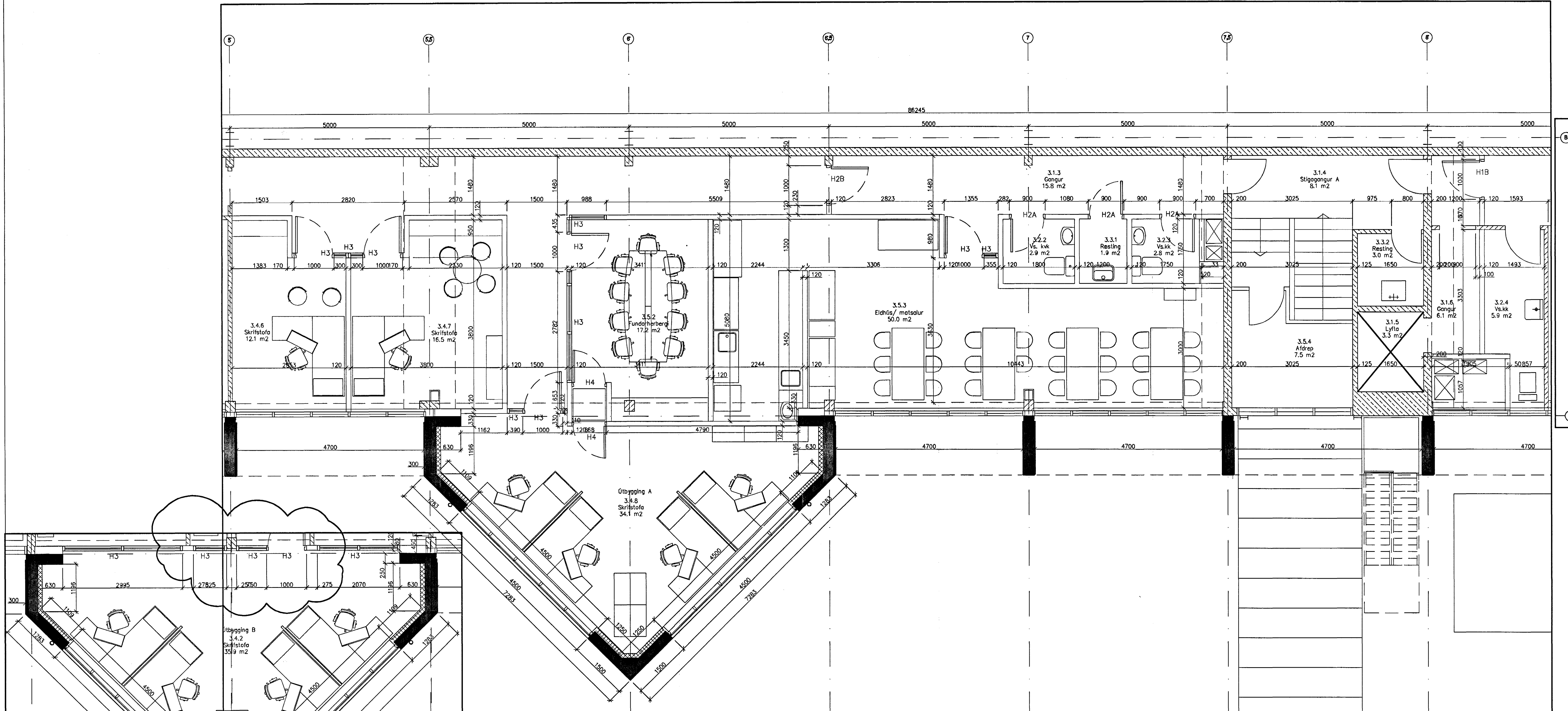
(99)3.07 Grunnmynd 3.hæð - Skrifstofuálm (partur) - mótuneyti
