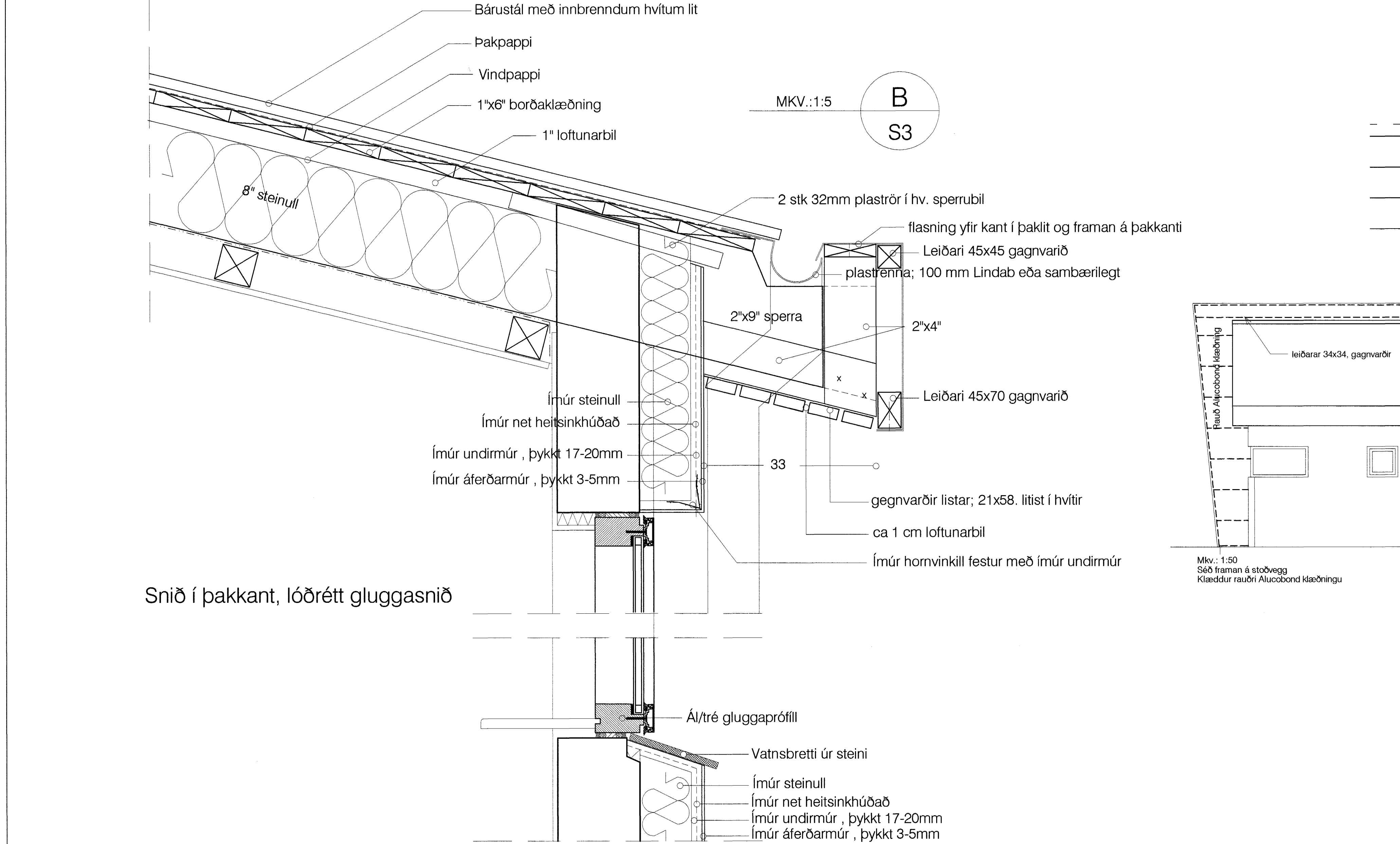
Snið í stoðvegg og þak
