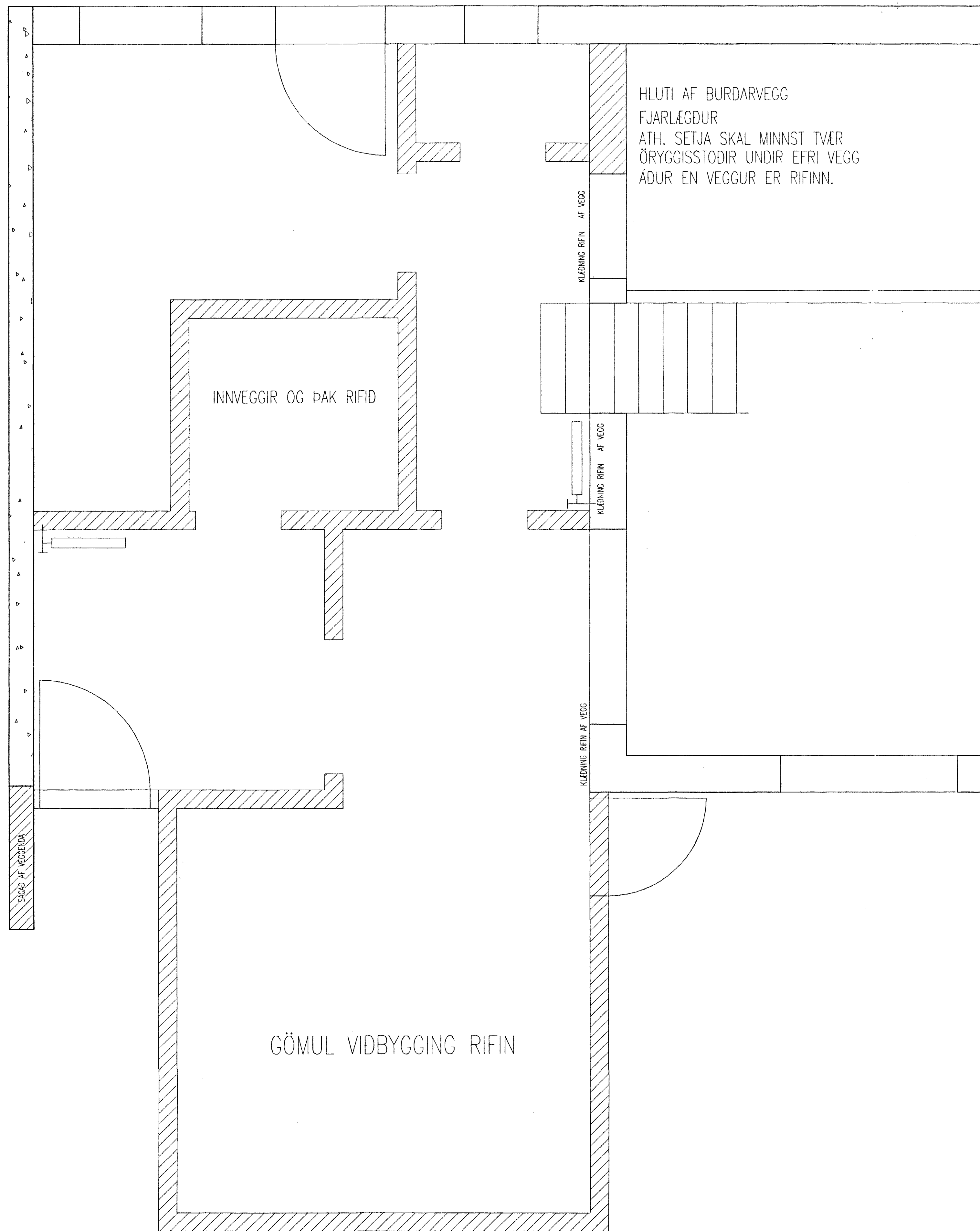
RIF VIÐBYGGINGAR OG INNVEGGJA, 1:20
