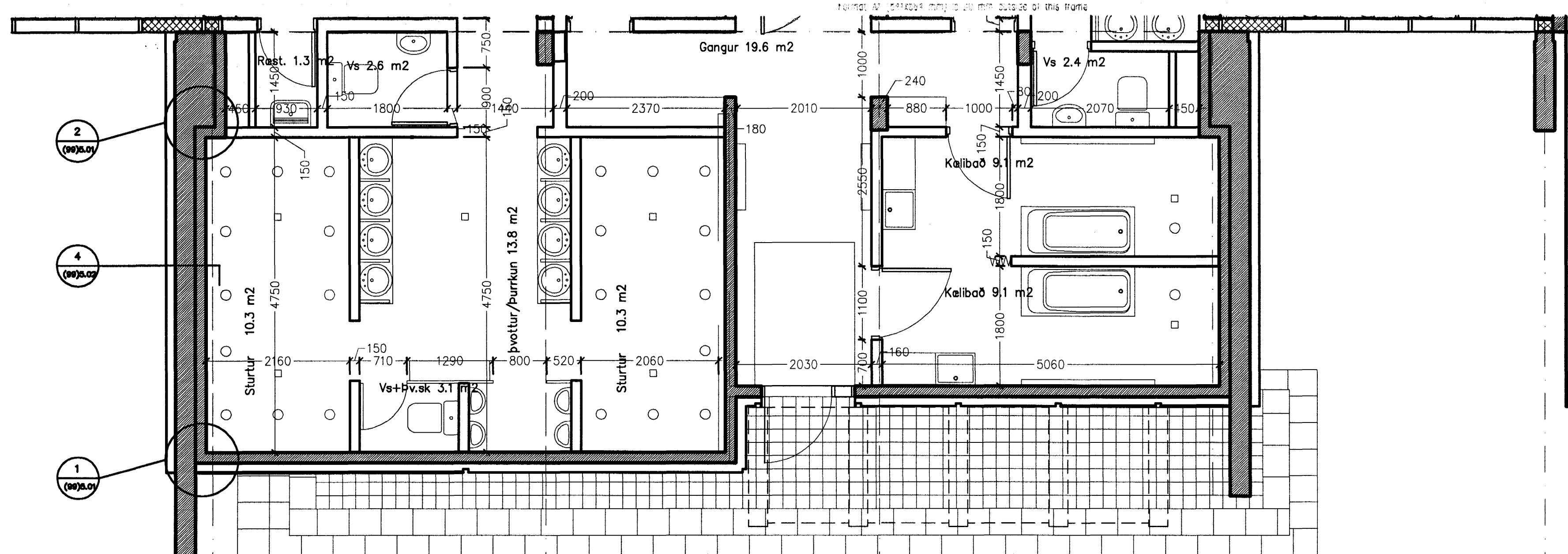
Baðhús, grunnmynd
