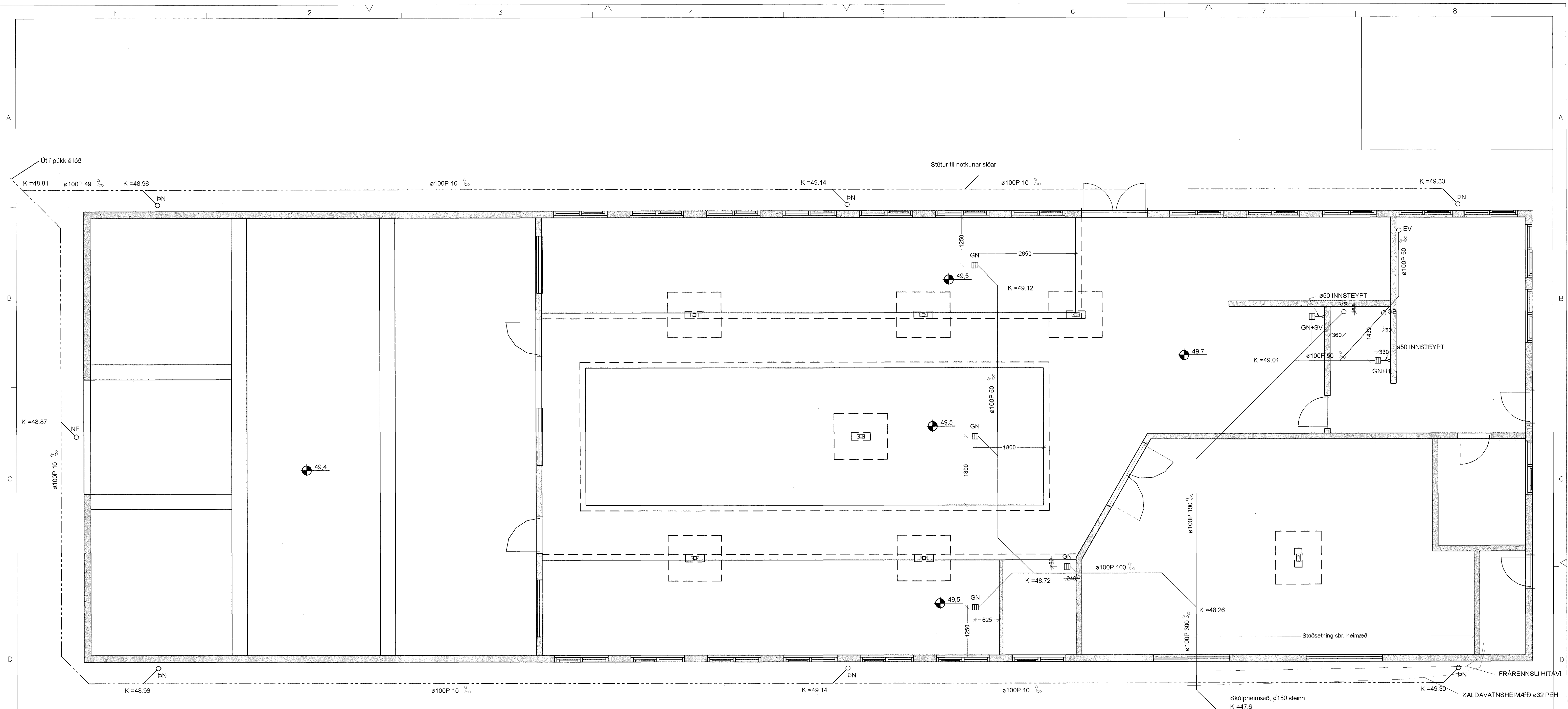
GRUNNMYND FRÁRENNSLISLAGNA. 1:50
