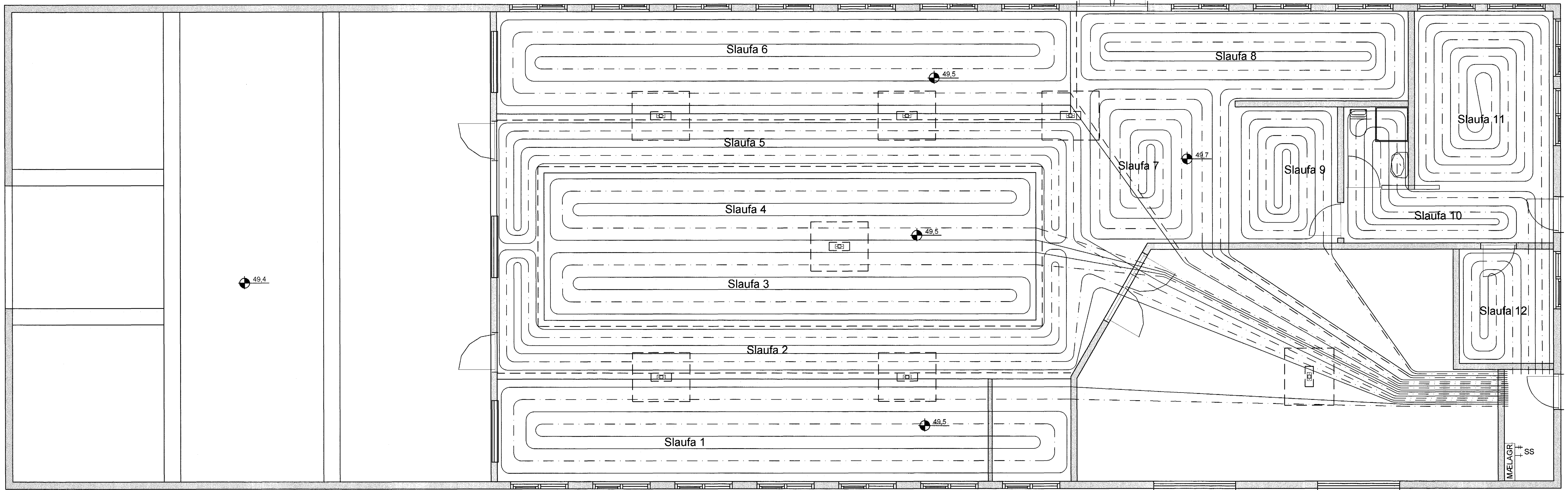
GRUNNMYND GÓLFHITALAGNA. 1:50
