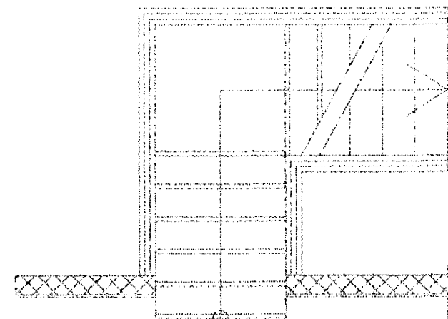
Gólfhitalagnir 1. hæð mkv. 1:50
