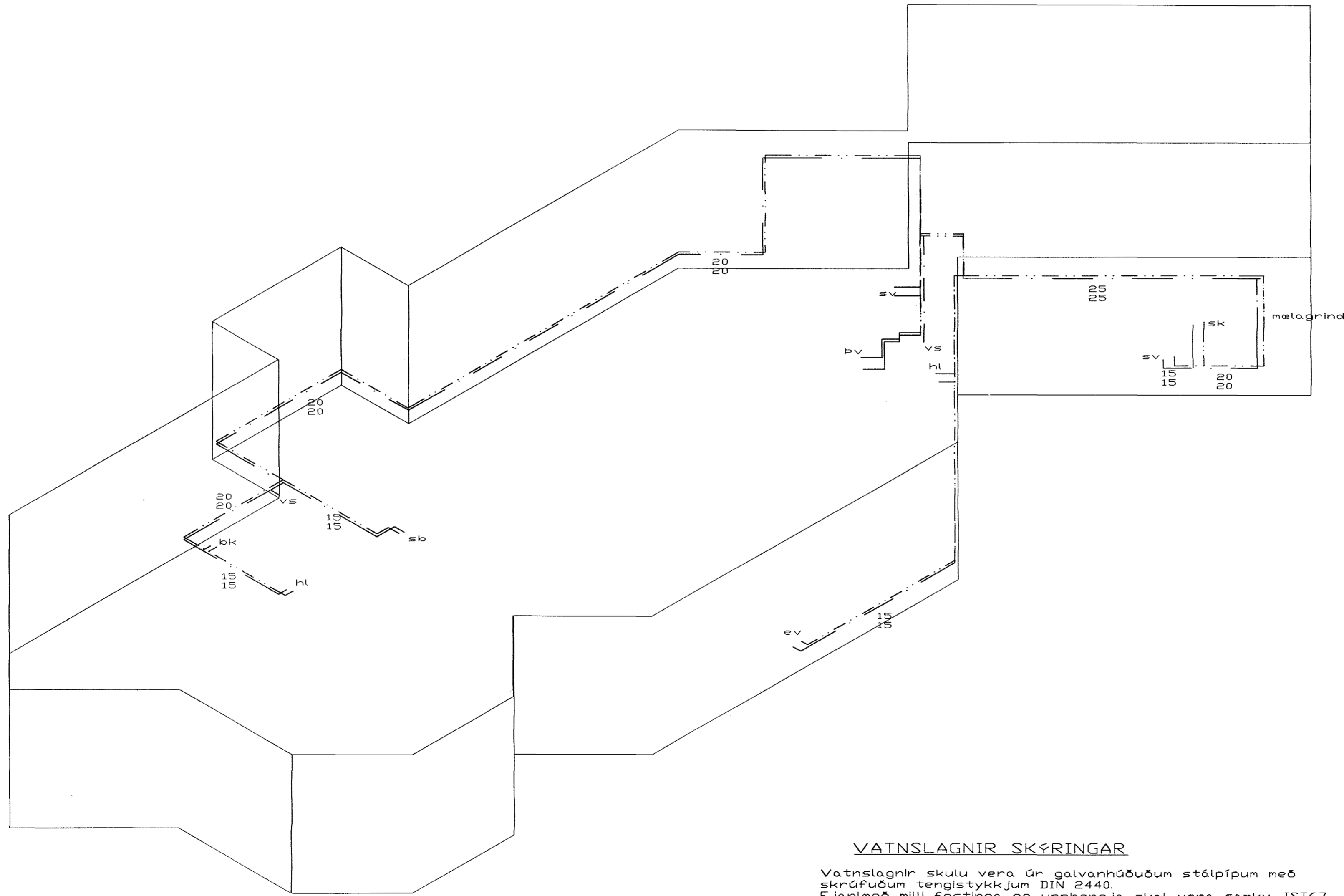
Rúmmynd vatnslagna ca 1/50
