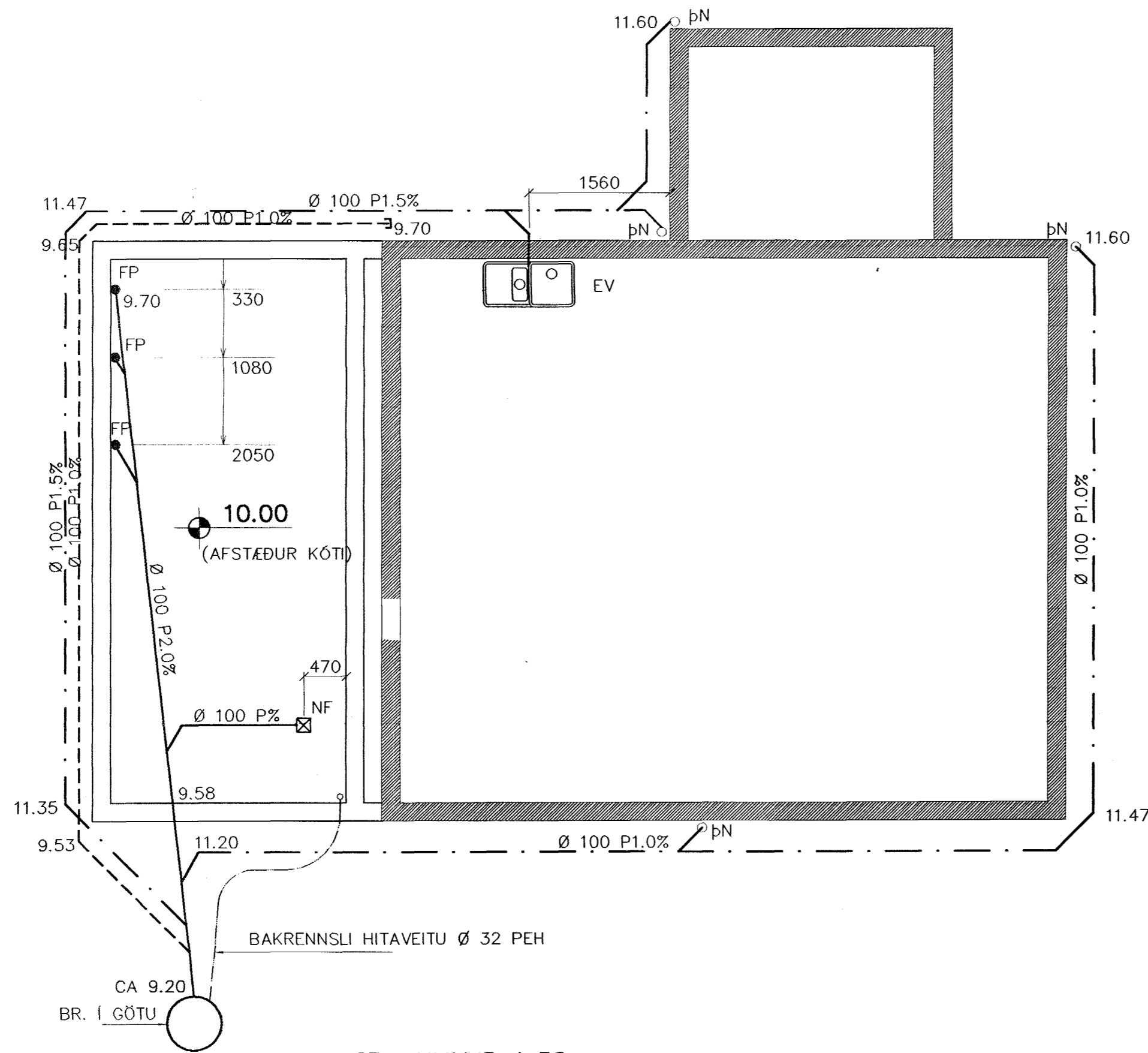
GRUNNMYND 1:50
