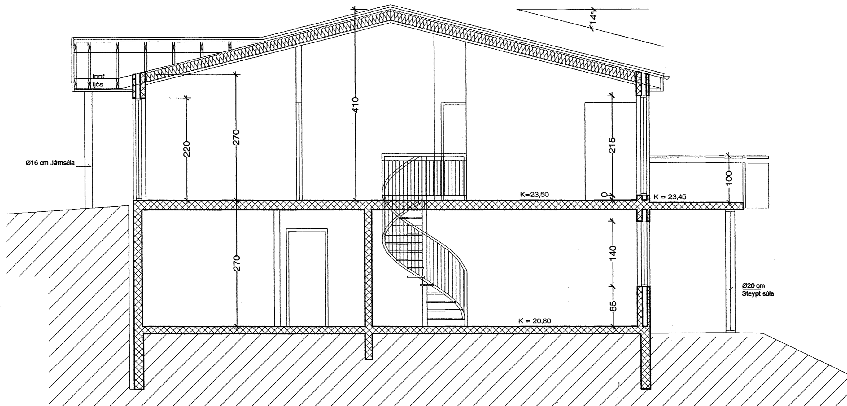
Sneiðing, 1:50
