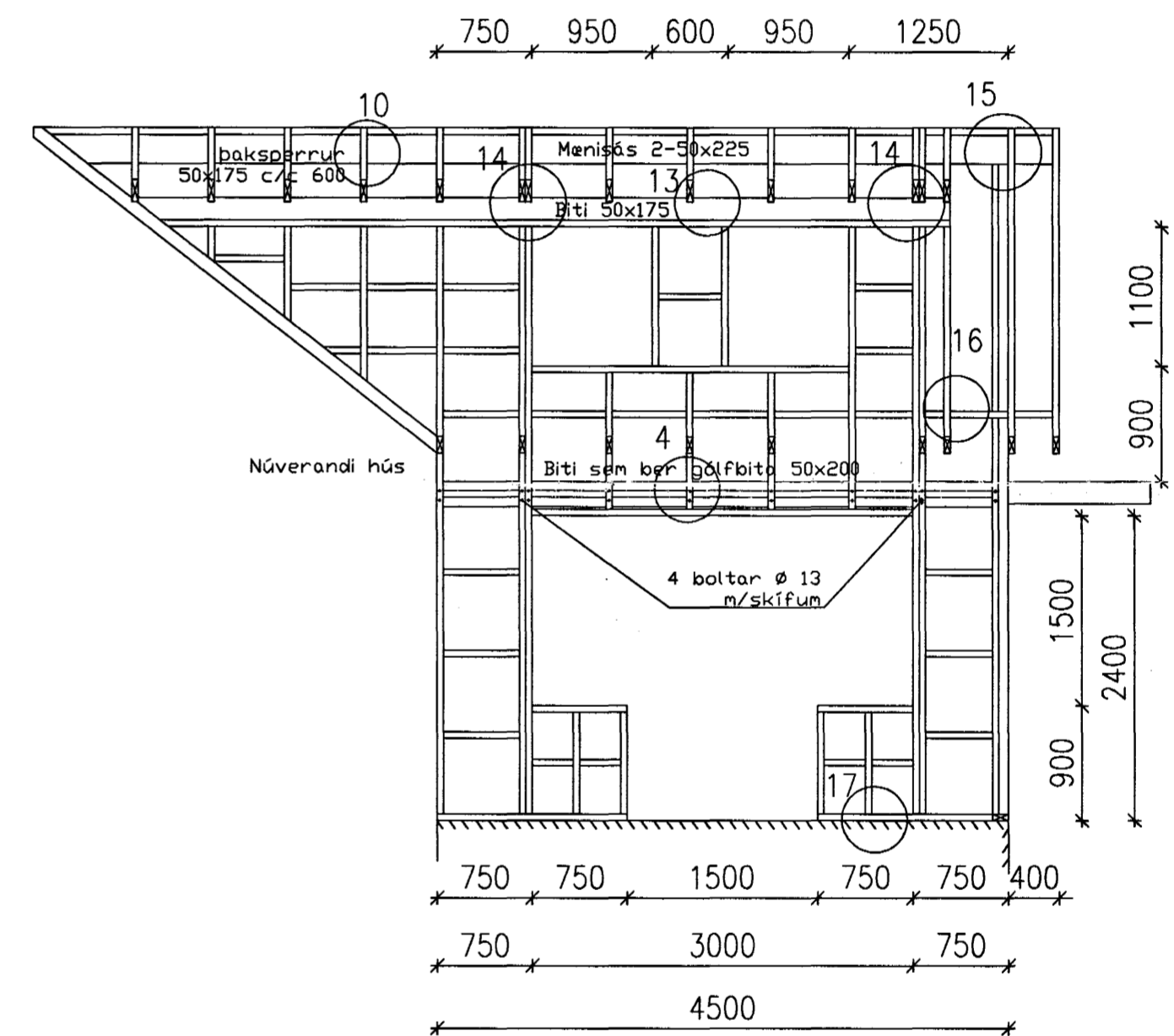
Vesturhlið
