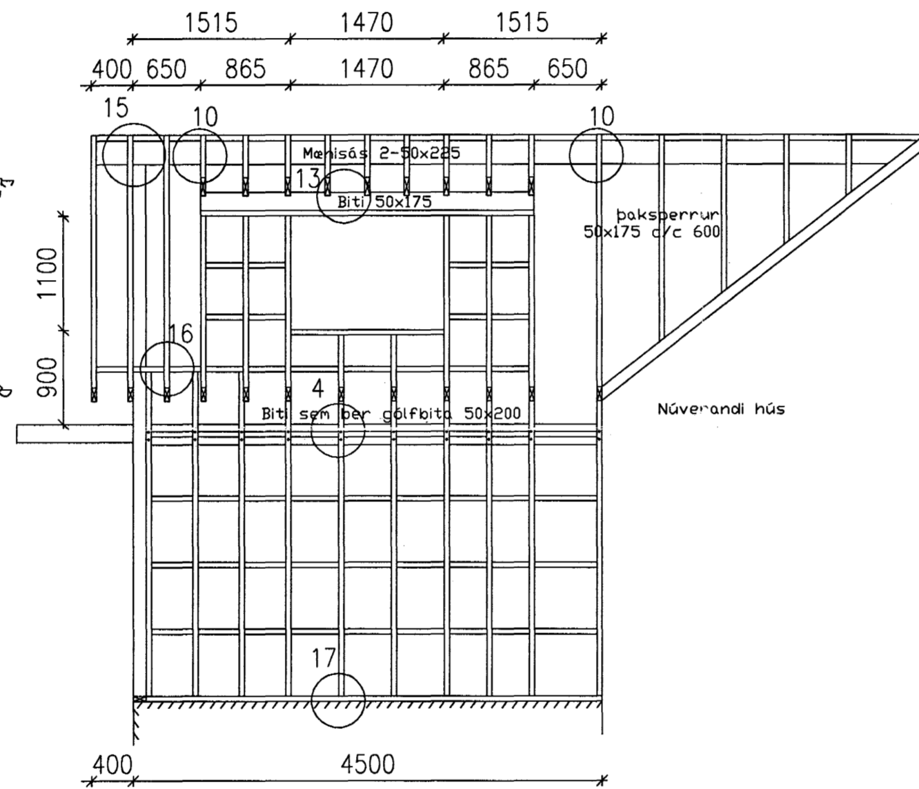
Austurhlið
