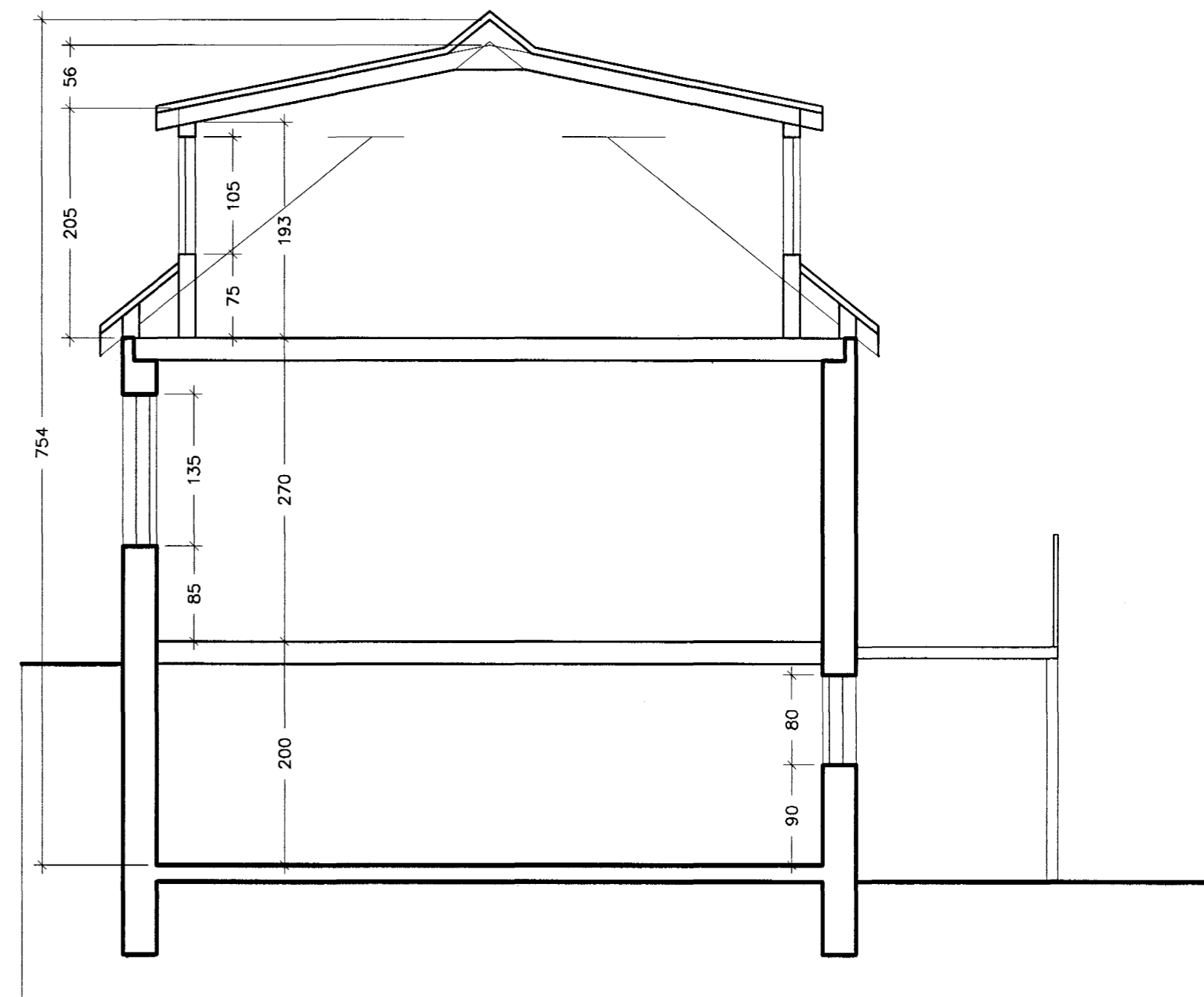
Sneiðing 1:50
