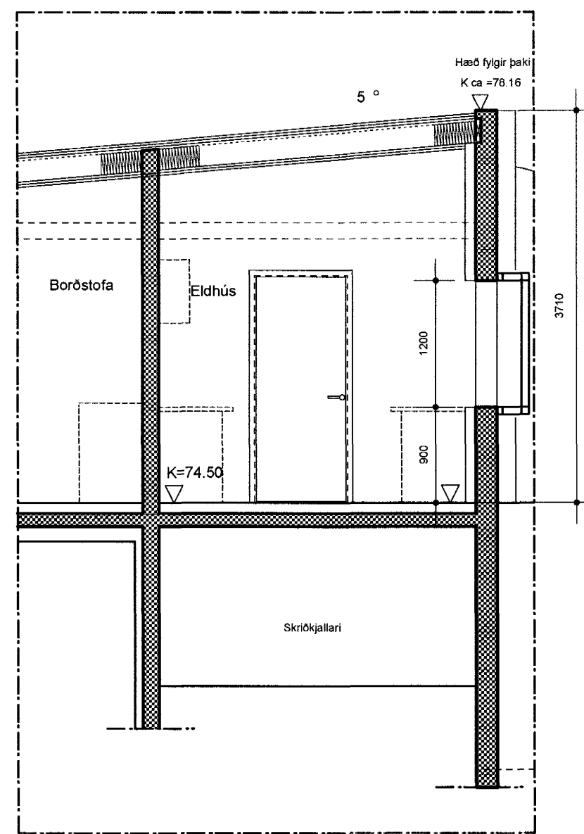
D-D Snið í eldhús 20-20 Mkv: 1:50
