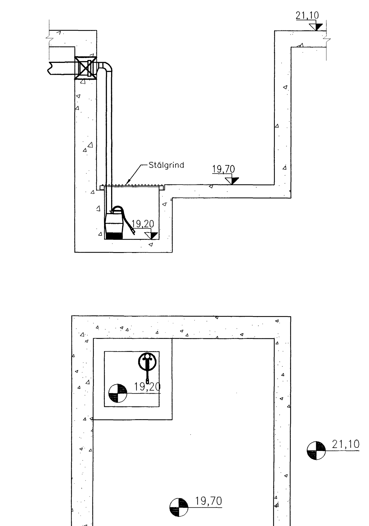
A Snið F-930 1:20
