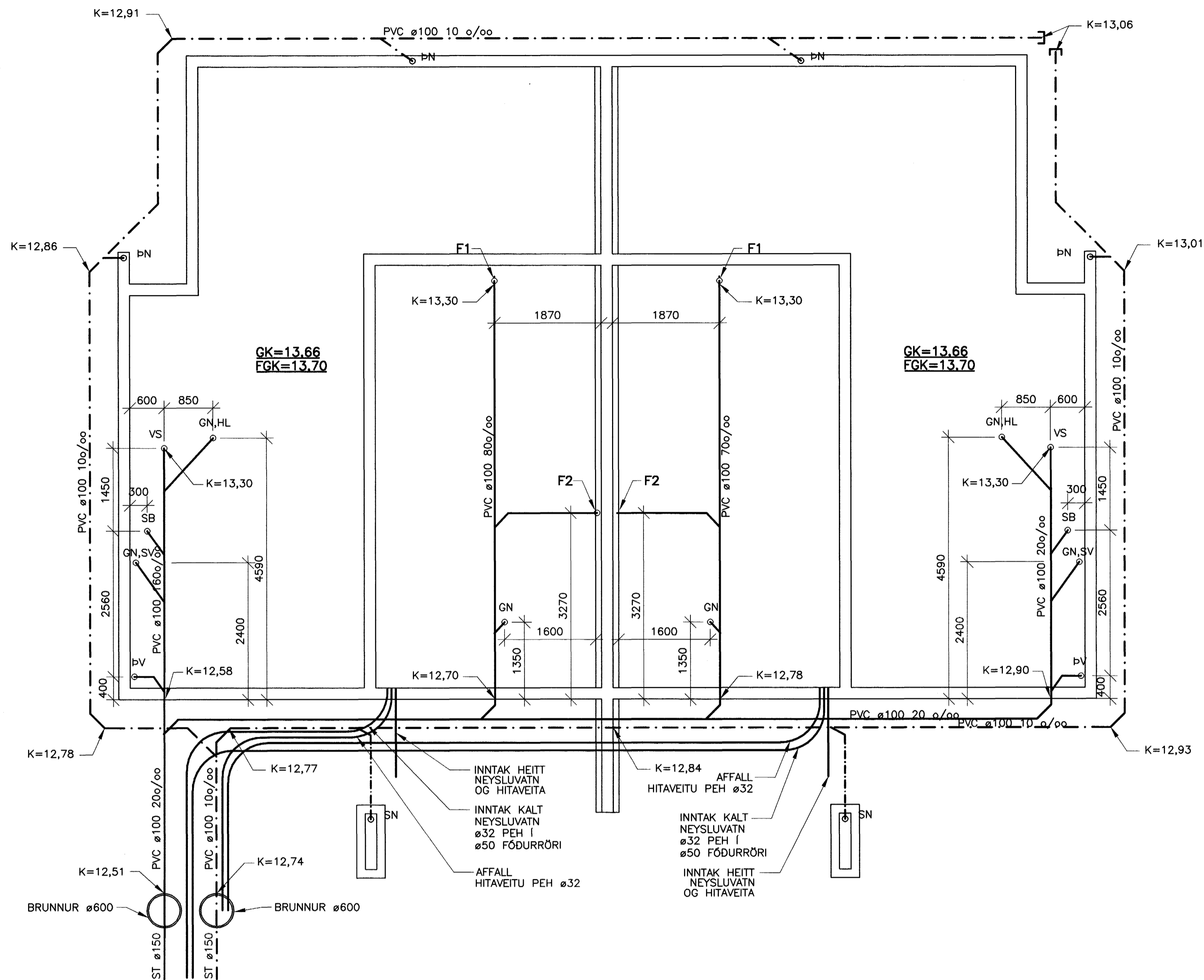
GRUNNLAGNIR GRUNNMÝND. 1:50
