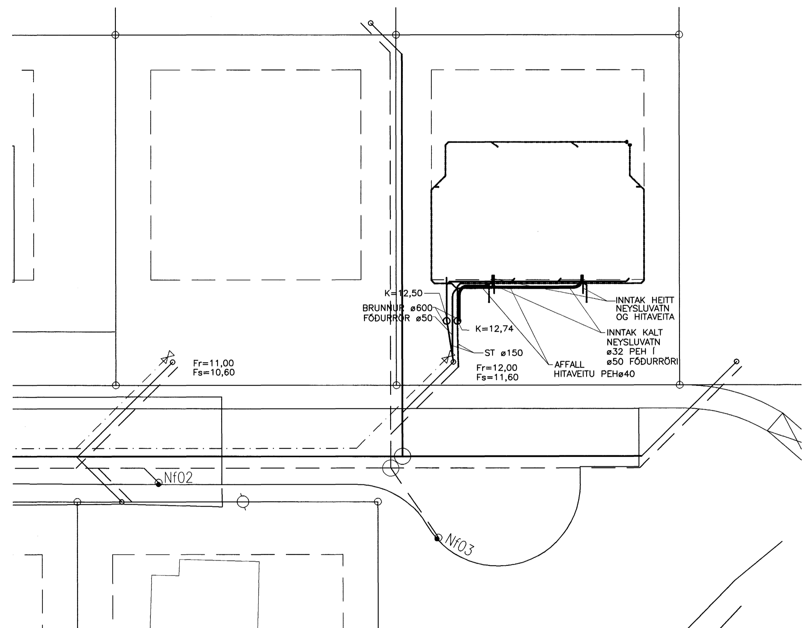
AFSTÖÐUMÝND. 1:200
