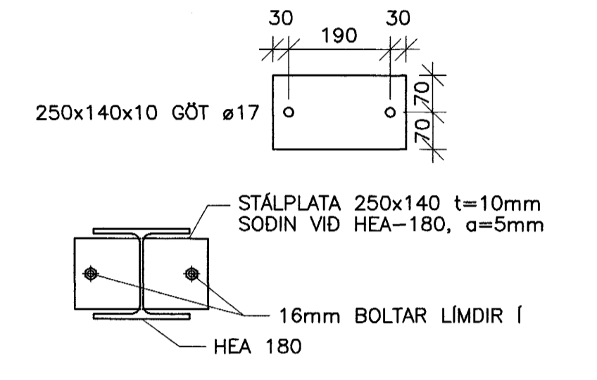
02 SNID, FESTING STÁLBITA VÍÐ VEGG 221 1:10
