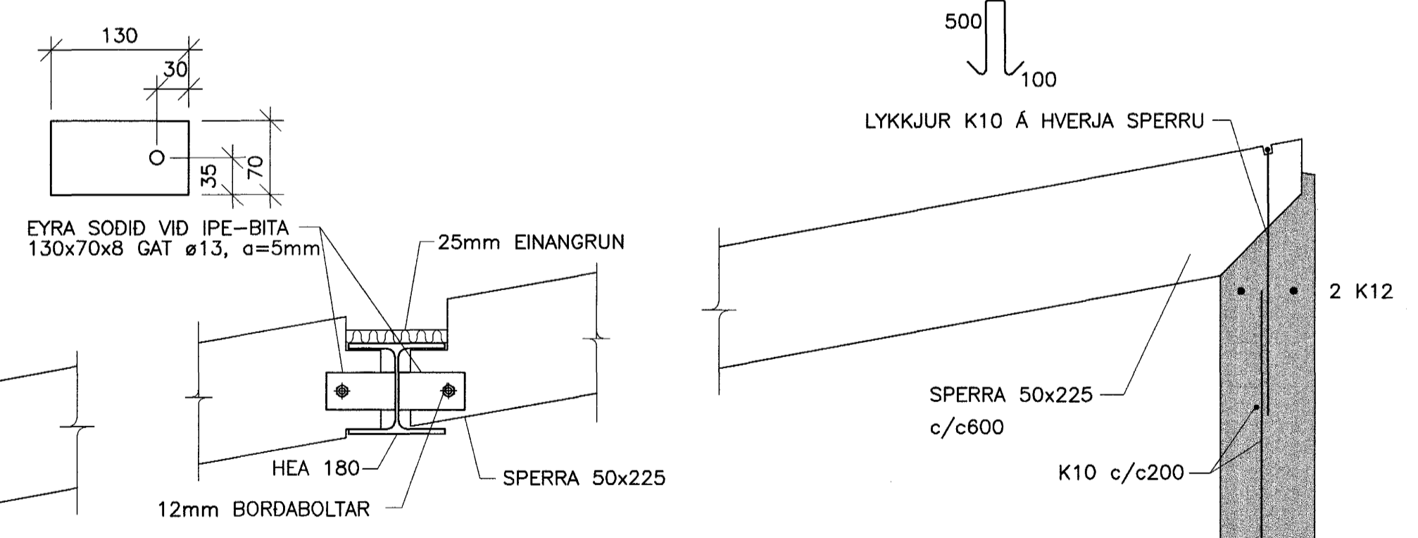
04 SNID, FESTING SPERRU VÍÐ STÁLBITA 221 1:10
