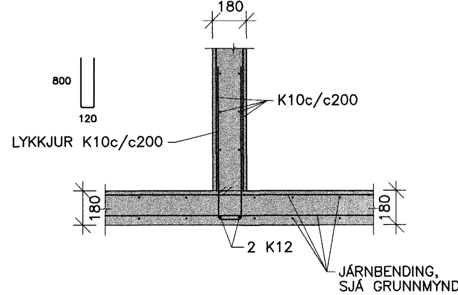
05 SNID 1:20
