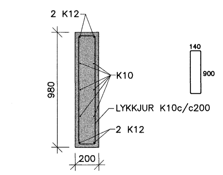
01 DEILI 1:20
