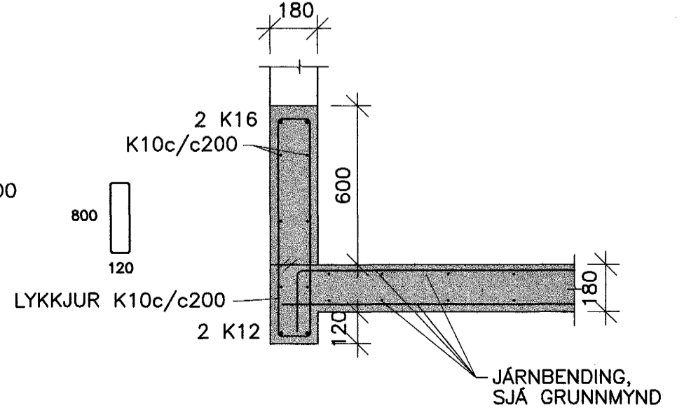
04 SNID 1:20
