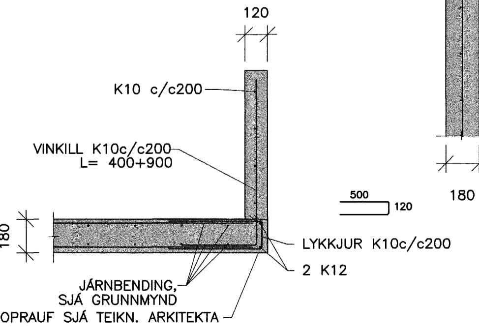
02 SNID 1:20
