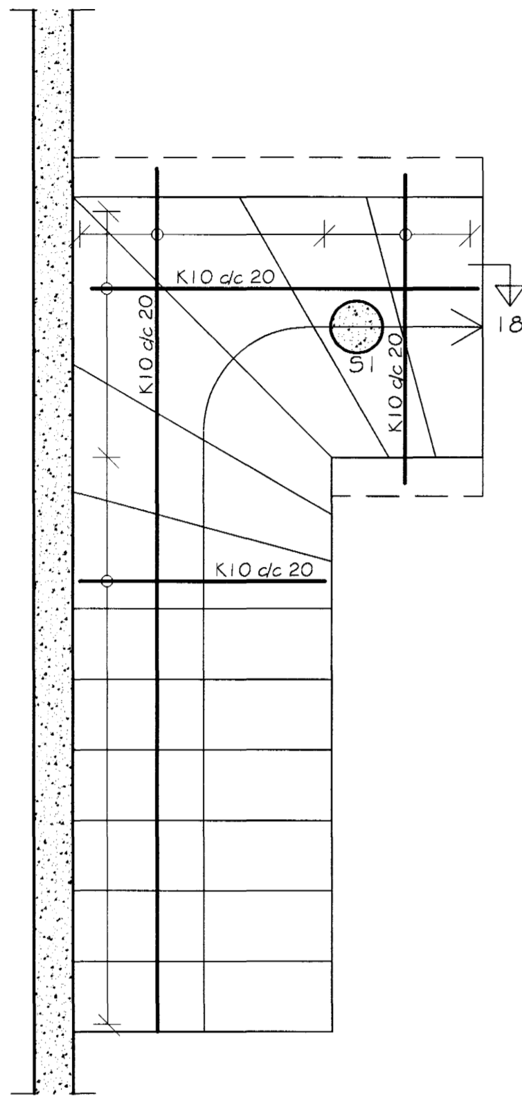
SVÖLUÁS 5 JÁRN Í STIGA MILLI HÆÐA GRUNNMYND MKV. 1:20
