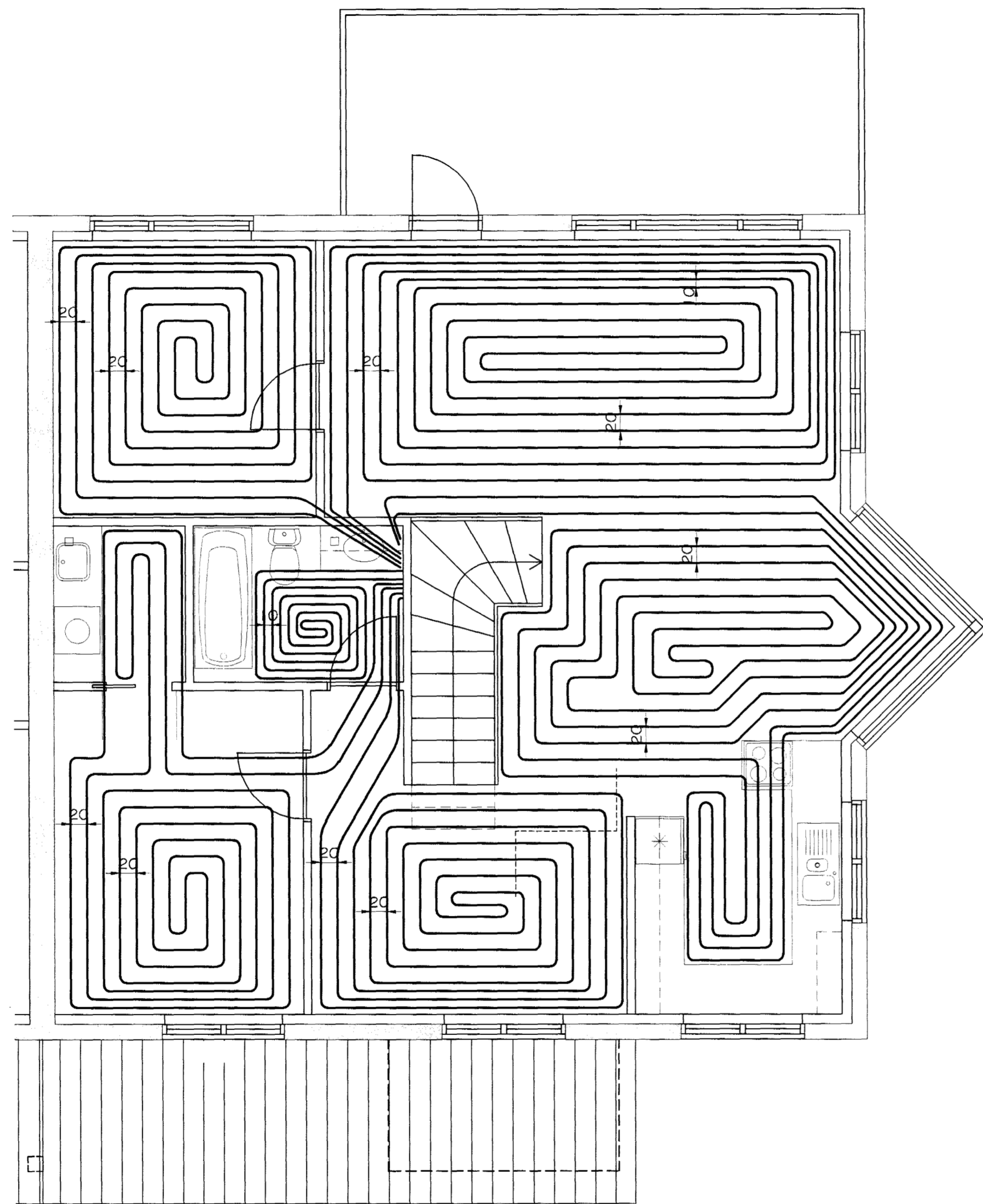
GÓLFHITALAGNIR GRUNNMYND EFRI HÆÐAR MKV. 1:50
