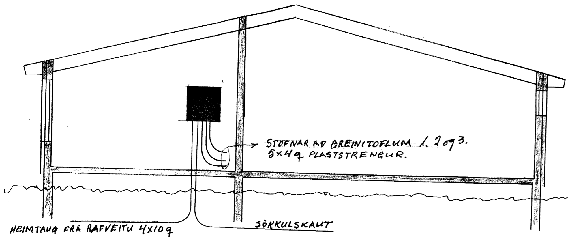
PVERSKURDUR A-A MAL 1:50
