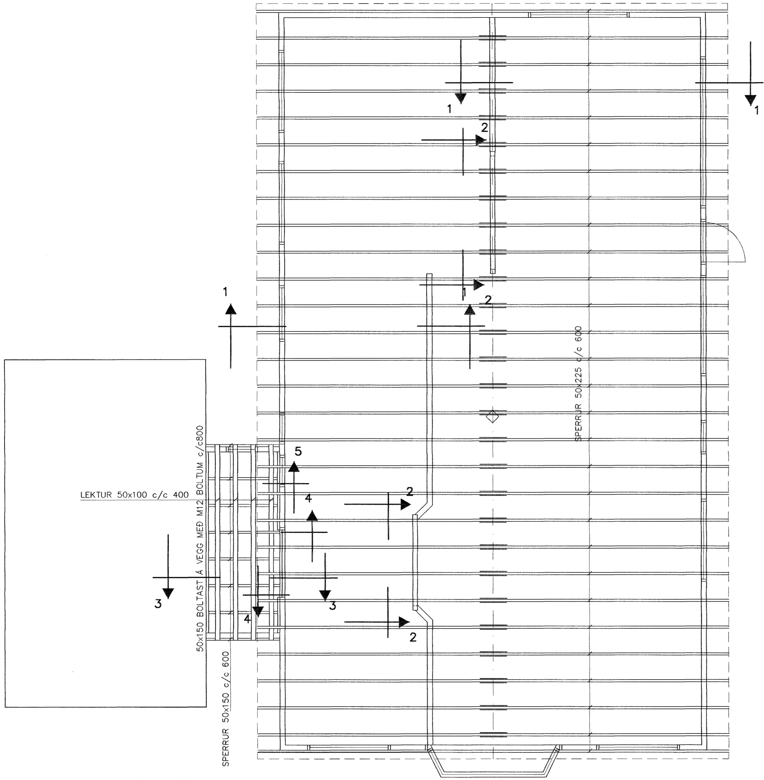
GRUNNMYND 1:50
