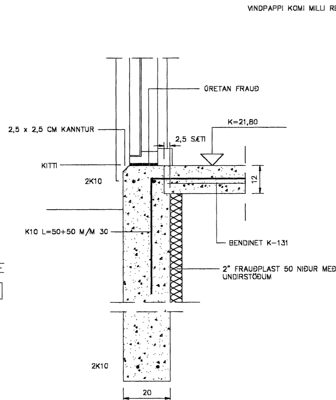
SNEIÐINGUR G, M=1:10
