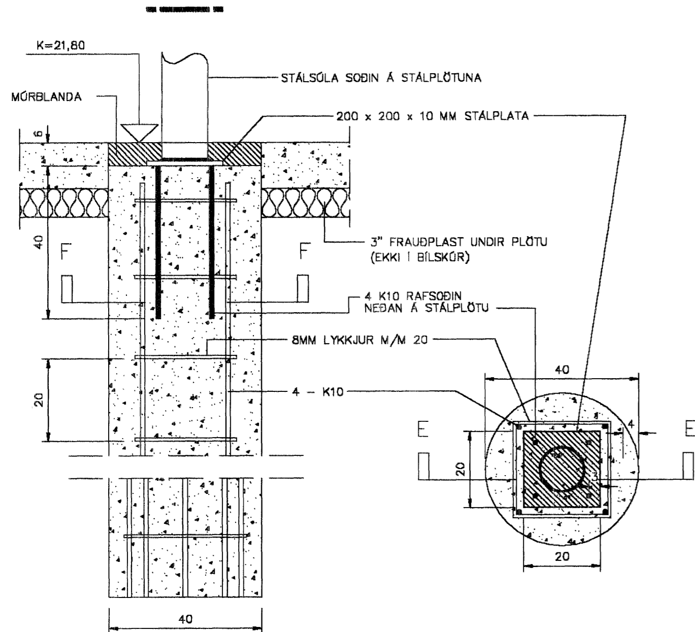
SNEIÐINGUR E, M=1:10
