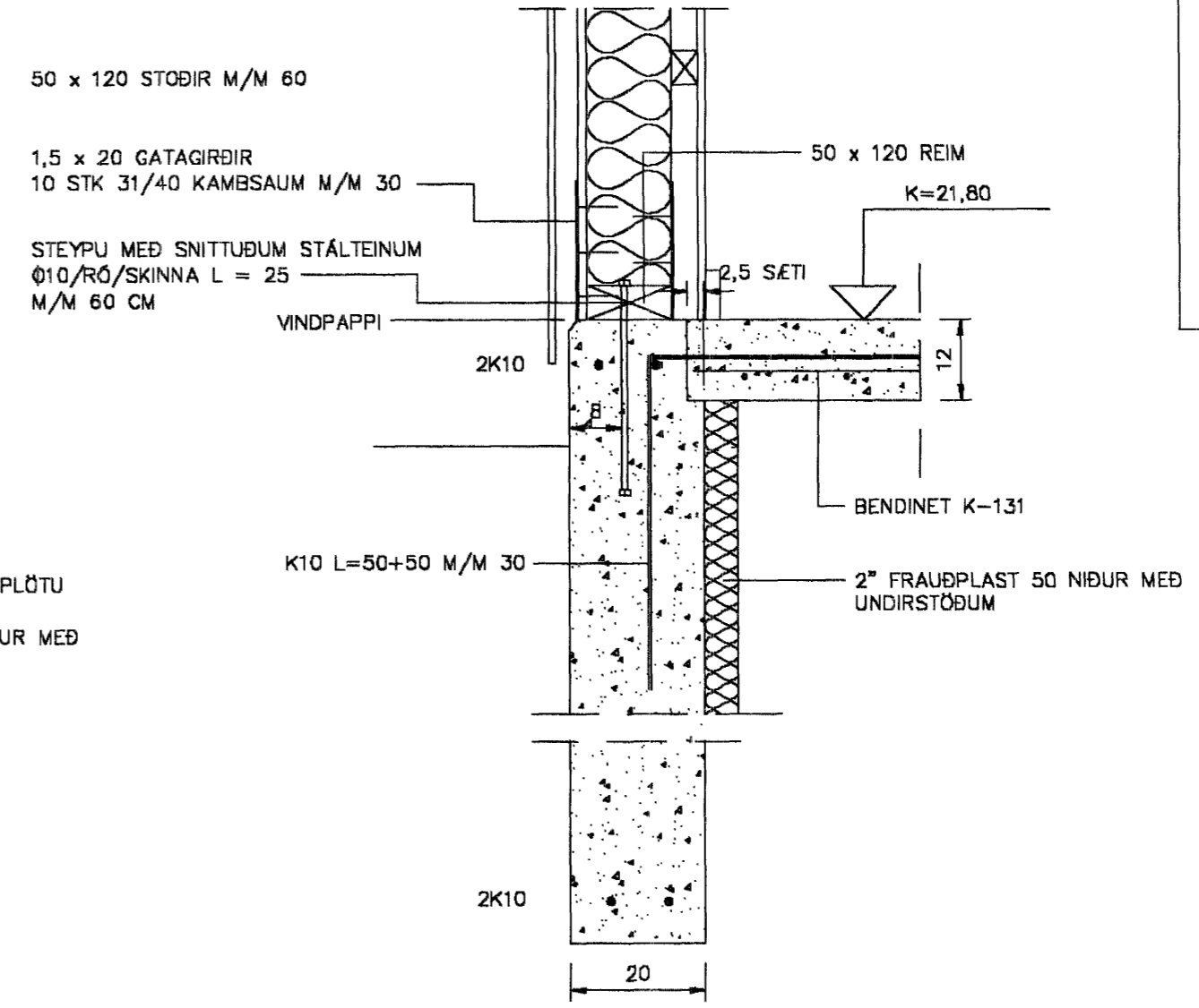
SNEIÐINGUR D, M=1:10
