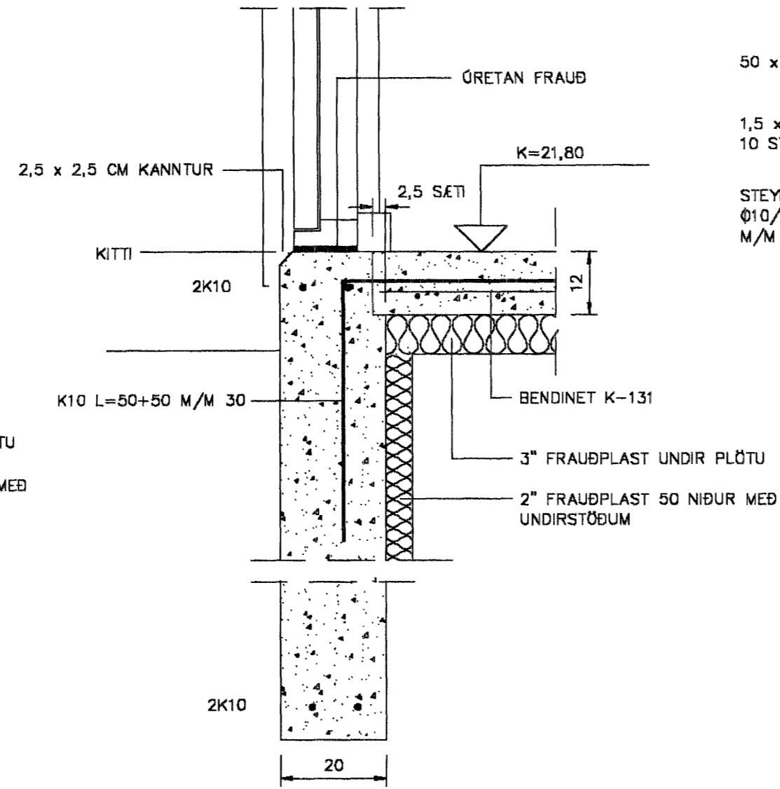
SNEIÐINGUR B, M=1:10
