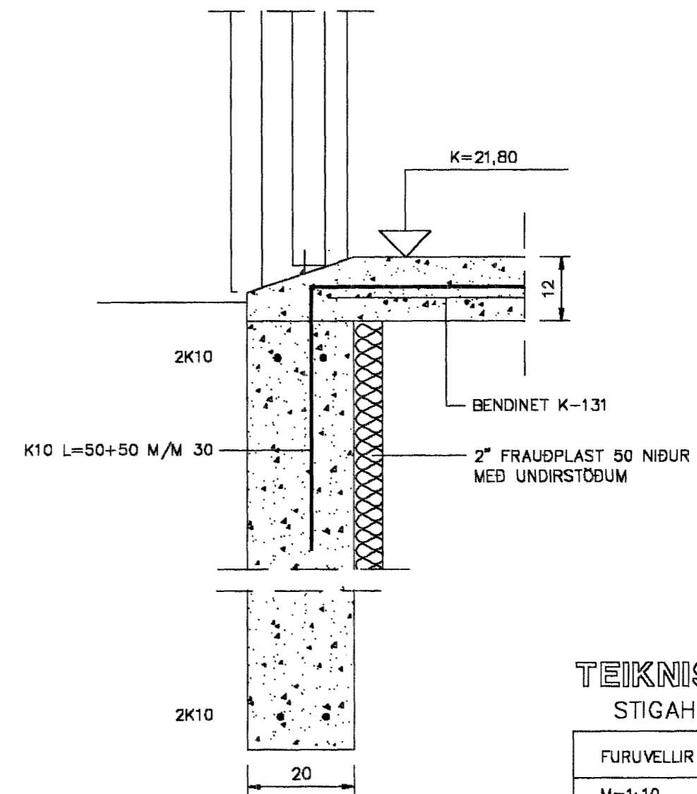
SNEIÐINGUR C, M=1:10
