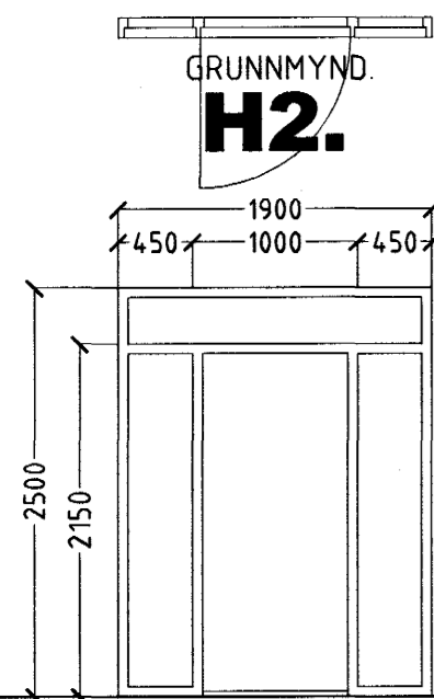
1 STK. ANDDYRI. HURÐ OPNAST VINSTRI ÚT.
