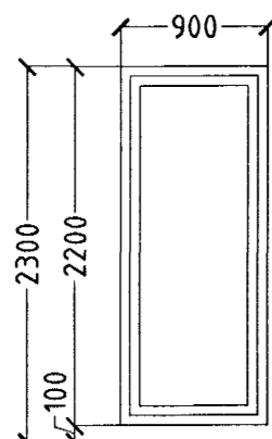
1 STK. BORDSTOFA. HURÐ OPNAST HÆGRI ÚT.
