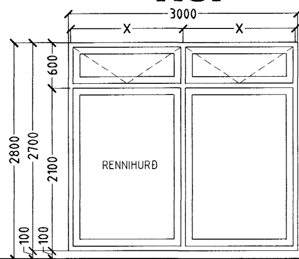
1 STK. STOFA. HURÐ ER RENNIHURÐ.
