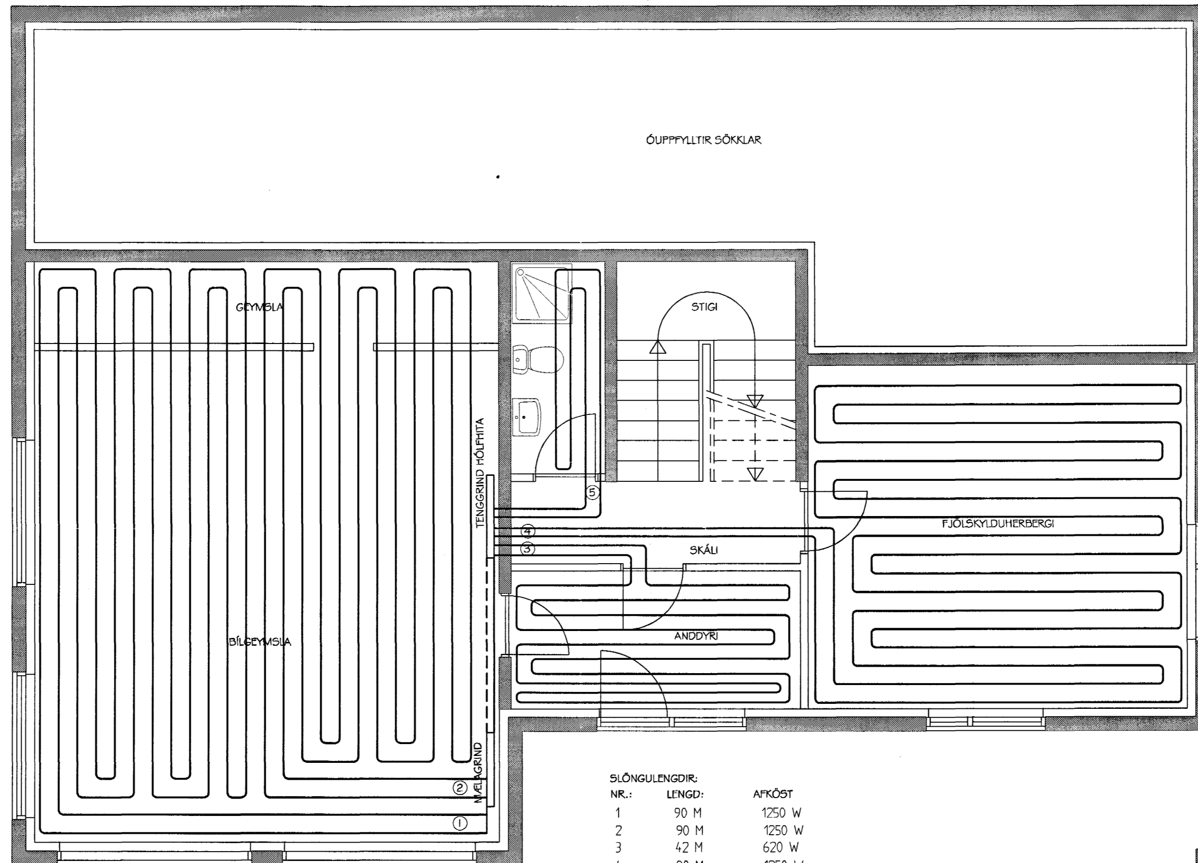
GÓLFHITALAGNIR GRUNNMYND NEDRI HÆÐAR MKV. 1:50
