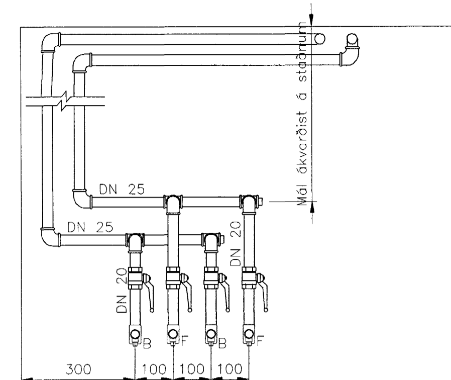
C Snið - í deilirör á útvegg - 1:10
