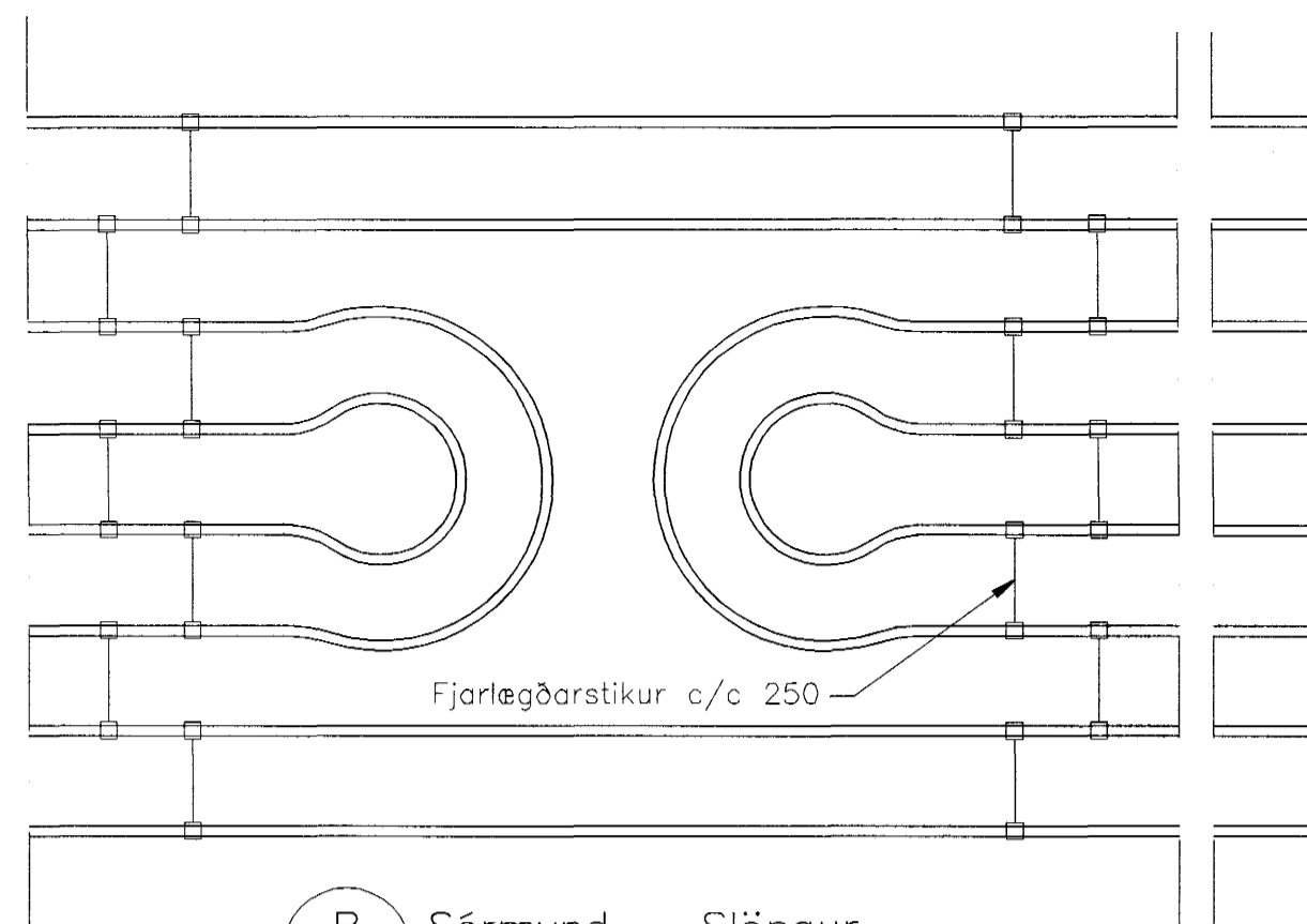
B Sérmynd - Slöngur - 1:20
