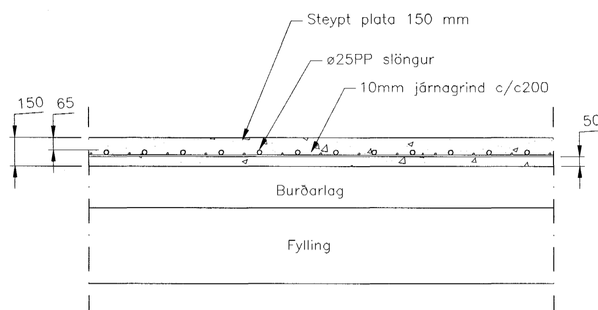
A Snið - slöngur í plötu - 1:20
