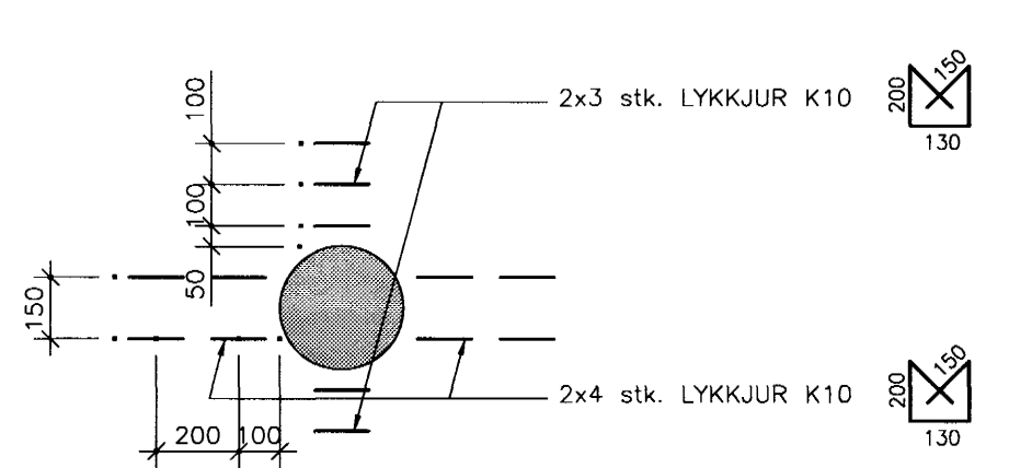
LYKKJUBENDING VID SÖLUR 1:20
