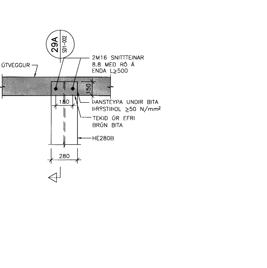
29A SNID 1:20
