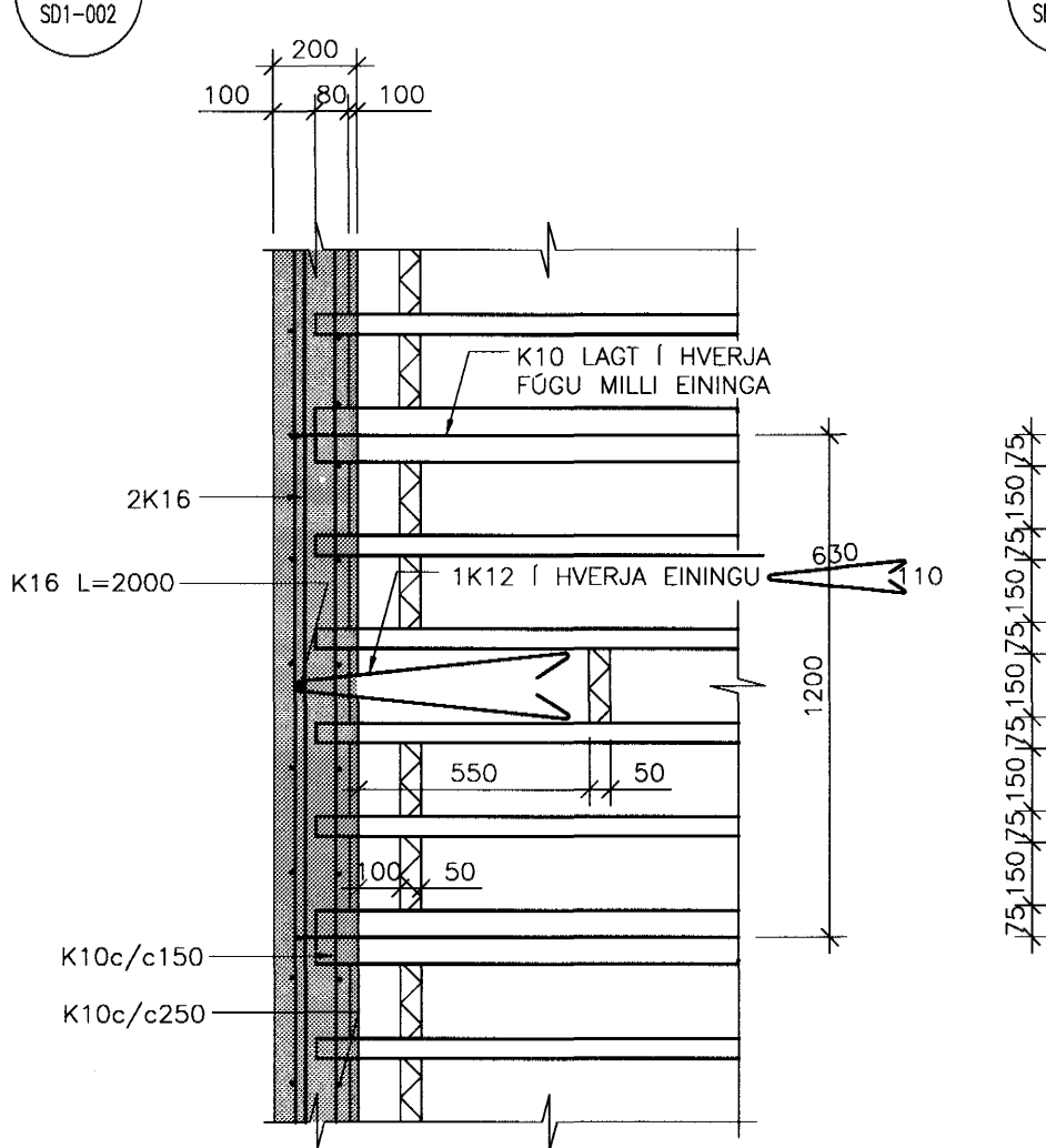
1A SNID 1:20
