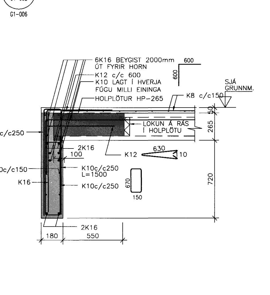
SM2 SÉRMYND 1:20
