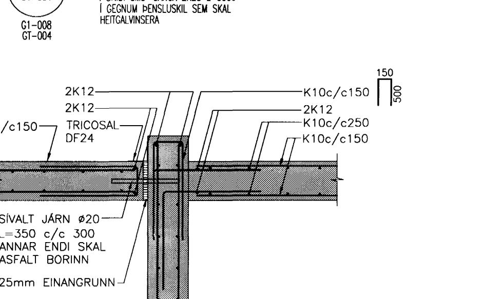
SM3 SÉRMYND 1:20
