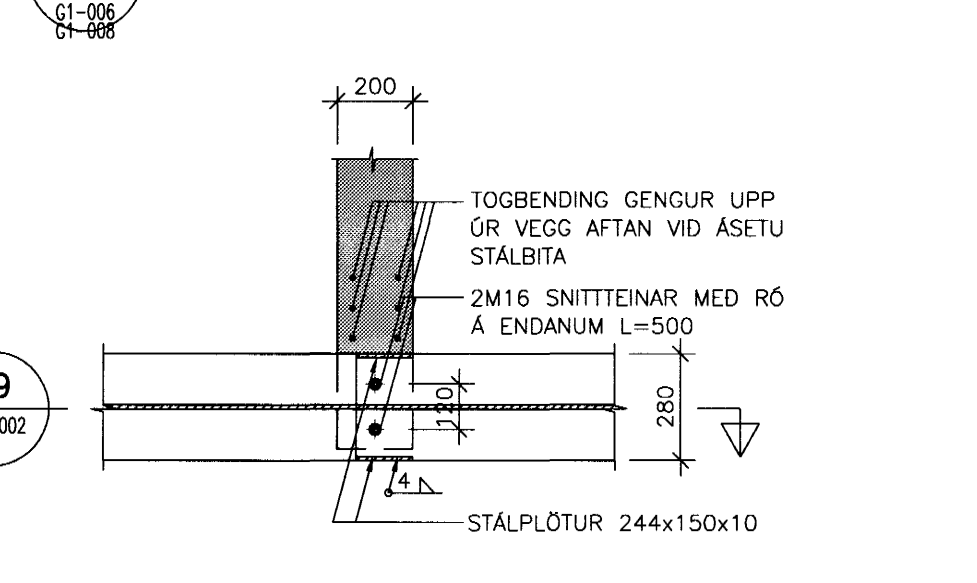
SM4 SÉRMYND 1:20
