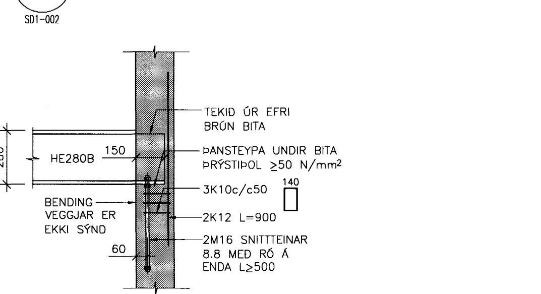
29A SNID 1:20
