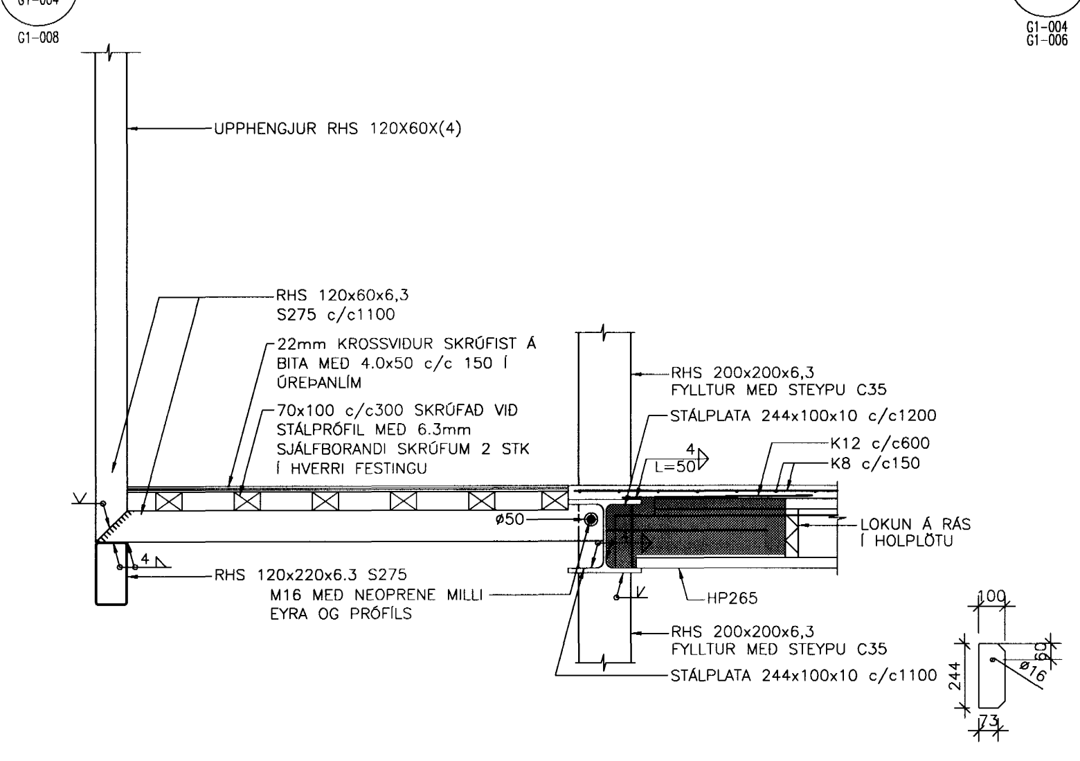
SM3 SÉRMYND 1:20
