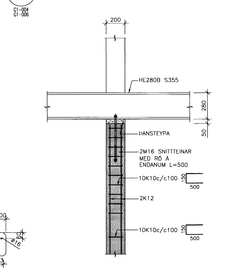
SM4 SÉRMYND 1:20
