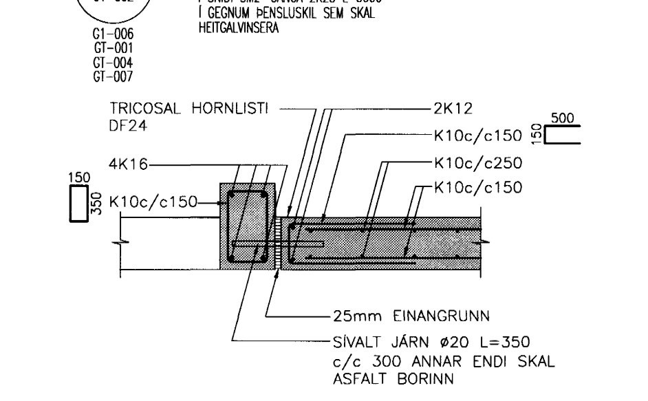
SM2 SÉRMYND 1:20
